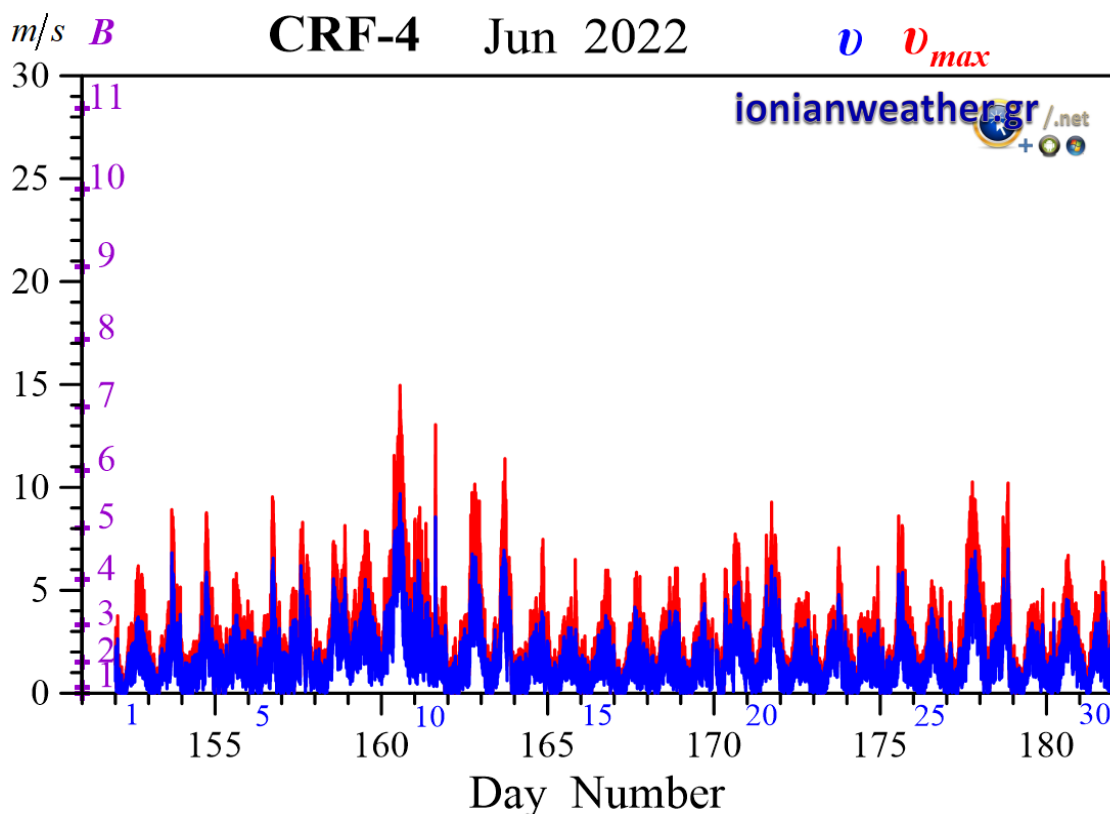
Εικόνα CRF4-2: Μέση ανά λεπτό ταχύτητα ανέμου ( m/s , γαλάζιο) και ριπή ανέμου (κόκκινο) Ιουνίου 2022. Κλίμακα ταχυτήτων αριστερά σε m/s και Beaufort .
