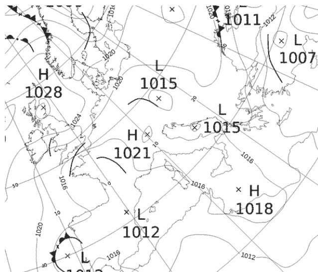
Εικόνα 3.1-4: MSLP 4 June 2022 00UTC
