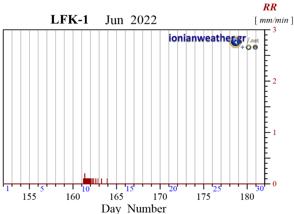
Εικόνα LFK1-1: Ανά λεπτό ρυθμός βροχόπτωσης (mm/min) Ιουνίου 2022.
