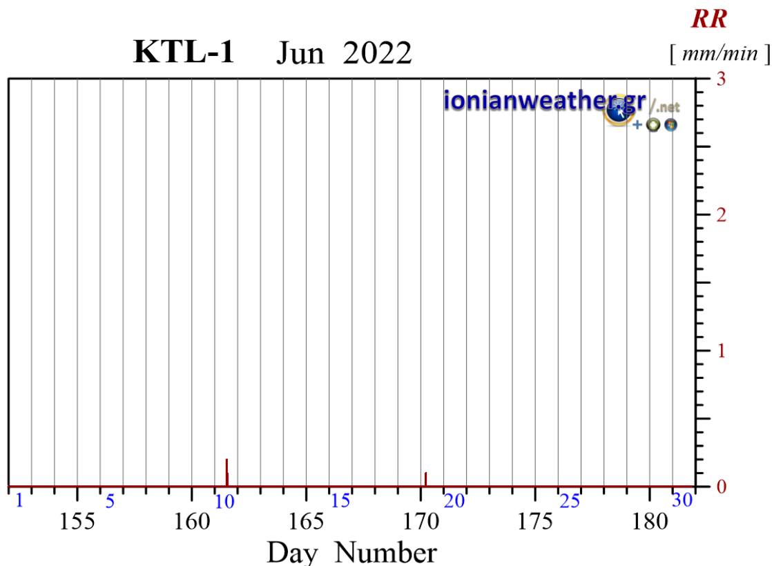
Εικόνα KTL1-1: Ανά λεπτό ρυθμός βροχόπτωσης (mm/min) Ιουνίου 2022.
