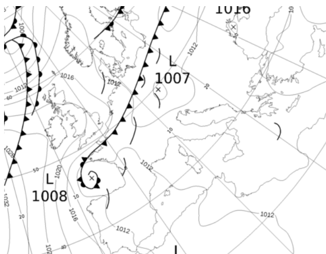
Εικόνα 3.1-21: MSLP 21 June 2022 00UTC
