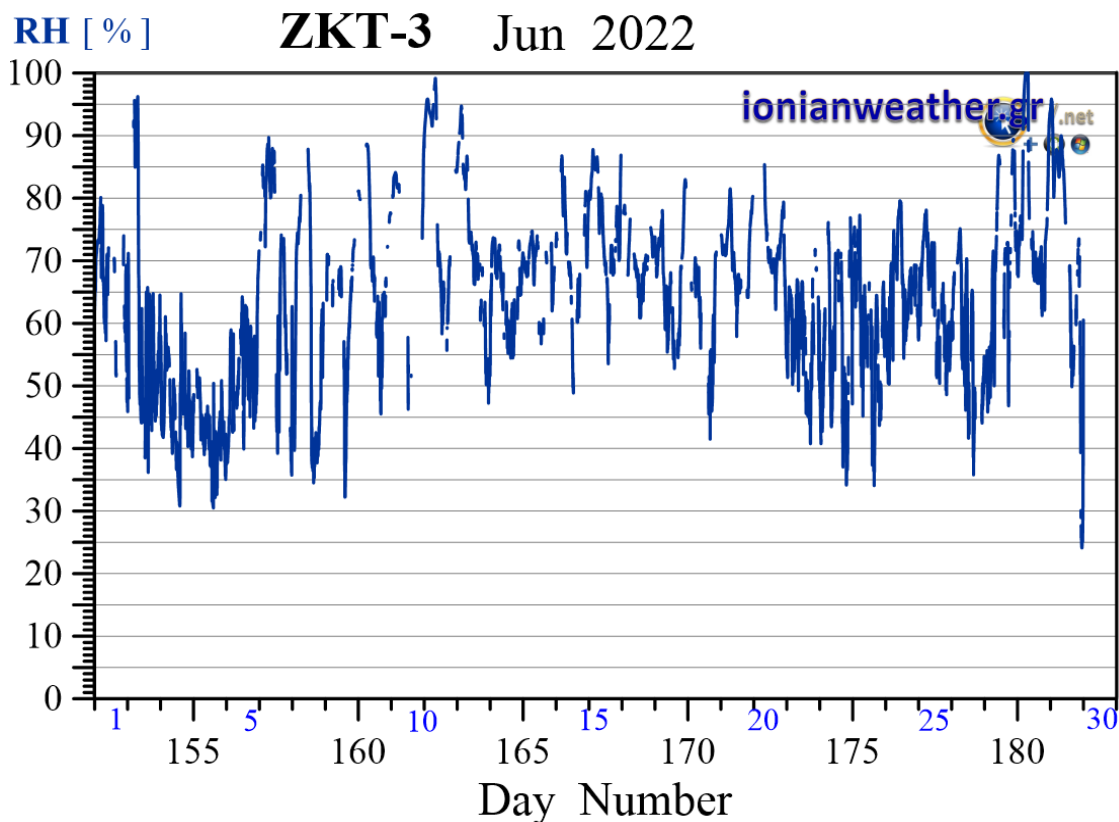
Εικόνα ZKT3-5: Μέση ανά λεπτό σχετική υγρασία Ιουνίου 2022.
