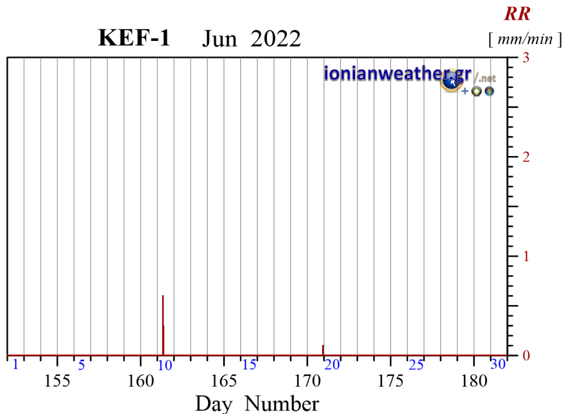
Εικόνα KEF1-1: Ανά λεπτό ρυθμός βροχόπτωσης (mm/min) Ιουνίου 2022.
