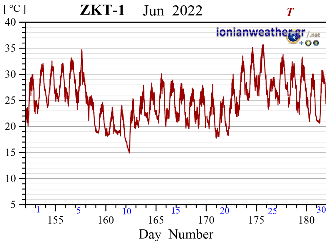
Εικόνα ZKT1-4: Μέση ανά λεπτό θερμοκρασία αέρα Ιουνίου 2022.
