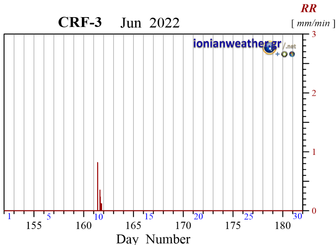
Εικόνα CRF3-1: Ανά λεπτό ρυθμός βροχόπτωσης (mm/min) Ιουνίου 2022.
