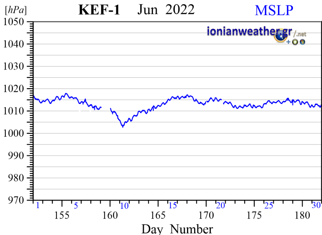
Εικόνα KEF1-6: Μέση ανά λεπτό βαρομετρική πίεση Ιουνίου 2022 ανηγμένη στην επιφάνεια της θάλασσας.
