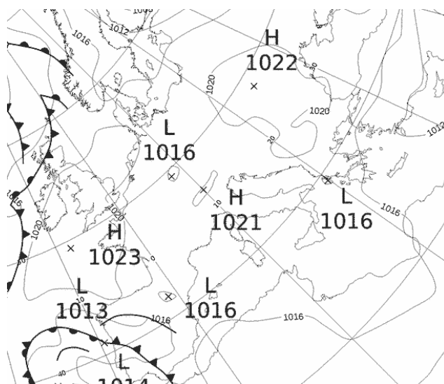
Εικόνα 3.1-16: MSLP 16 June 2022 00UTC
