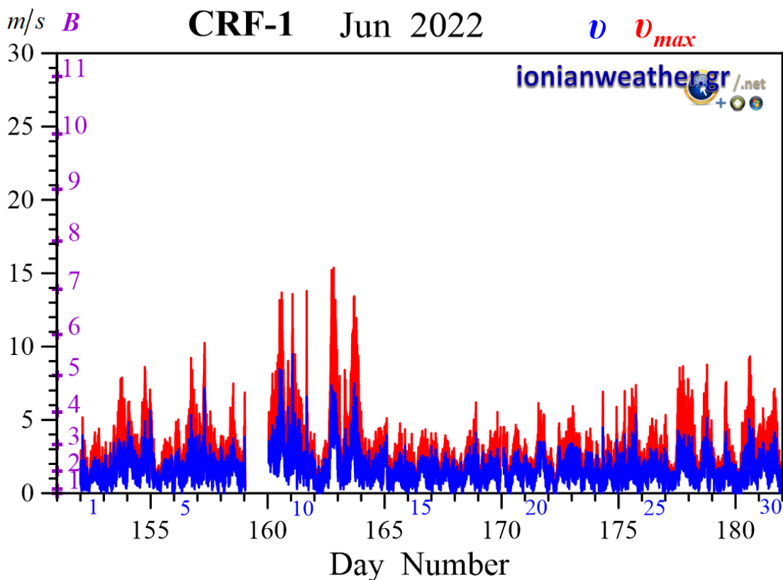
Εικόνα CRF1-2: Μέση ανά λεπτό ταχύτητα ανέμου ( m/s , γαλάζιο) και ριπή ανέμου (κόκκινο) Ιουνίου 2022. Κλίμακα ταχυτήτων αριστερά σε m/s και Beaufort.
