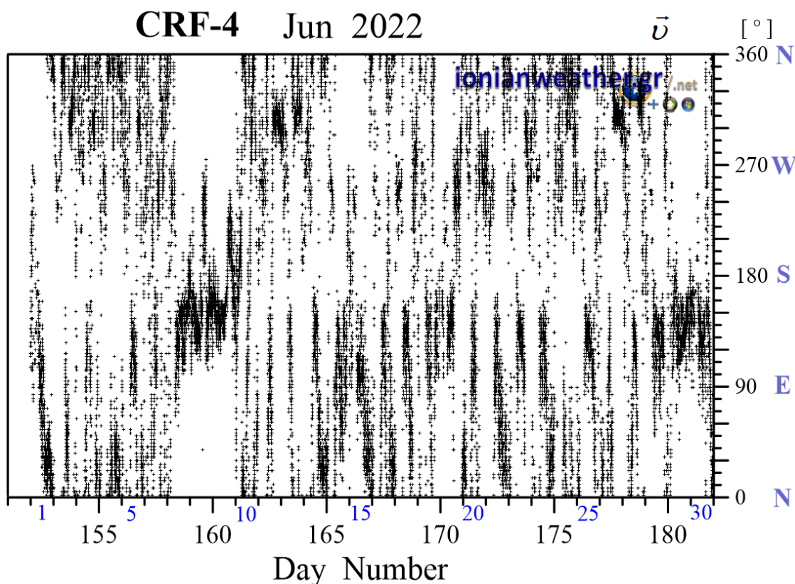
Εικόνα CRF4-3: Μέση ανά λεπτό κατεύθυνση ανέμου Ιουνίου 2022 (κλίμακα αζιμουθίων δεξιά)
