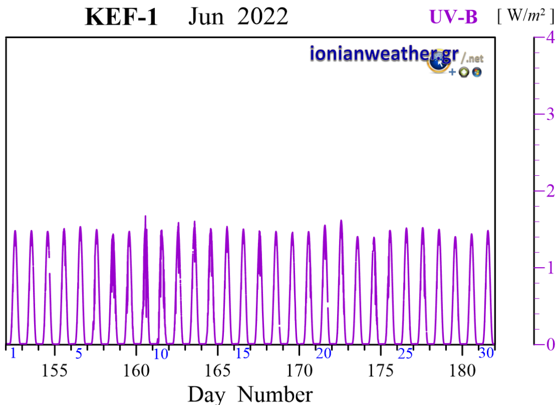
Εικόνα KEF1-9: Μέση ανά λεπτό Ηλιακή ακτινοβολία Ιουνίου 2022 στη φασματική περιοχή UVB
