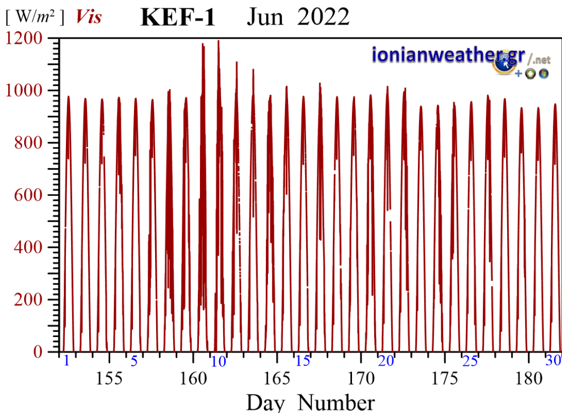
Εικόνα KEF1-7: Μέση ανά λεπτό Ηλιακή ακτινοβολία Ιουνίου 2022 στην οπτική και εγγύς υπέρυθρη περιοχή.
