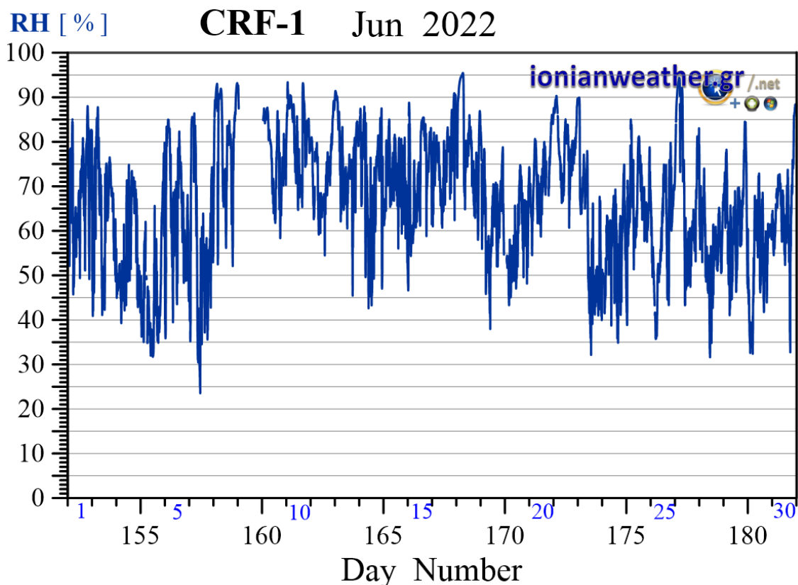
Εικόνα CRF1-5: Μέση ανά λεπτό σχετική υγρασία Ιουνίου 2022.
