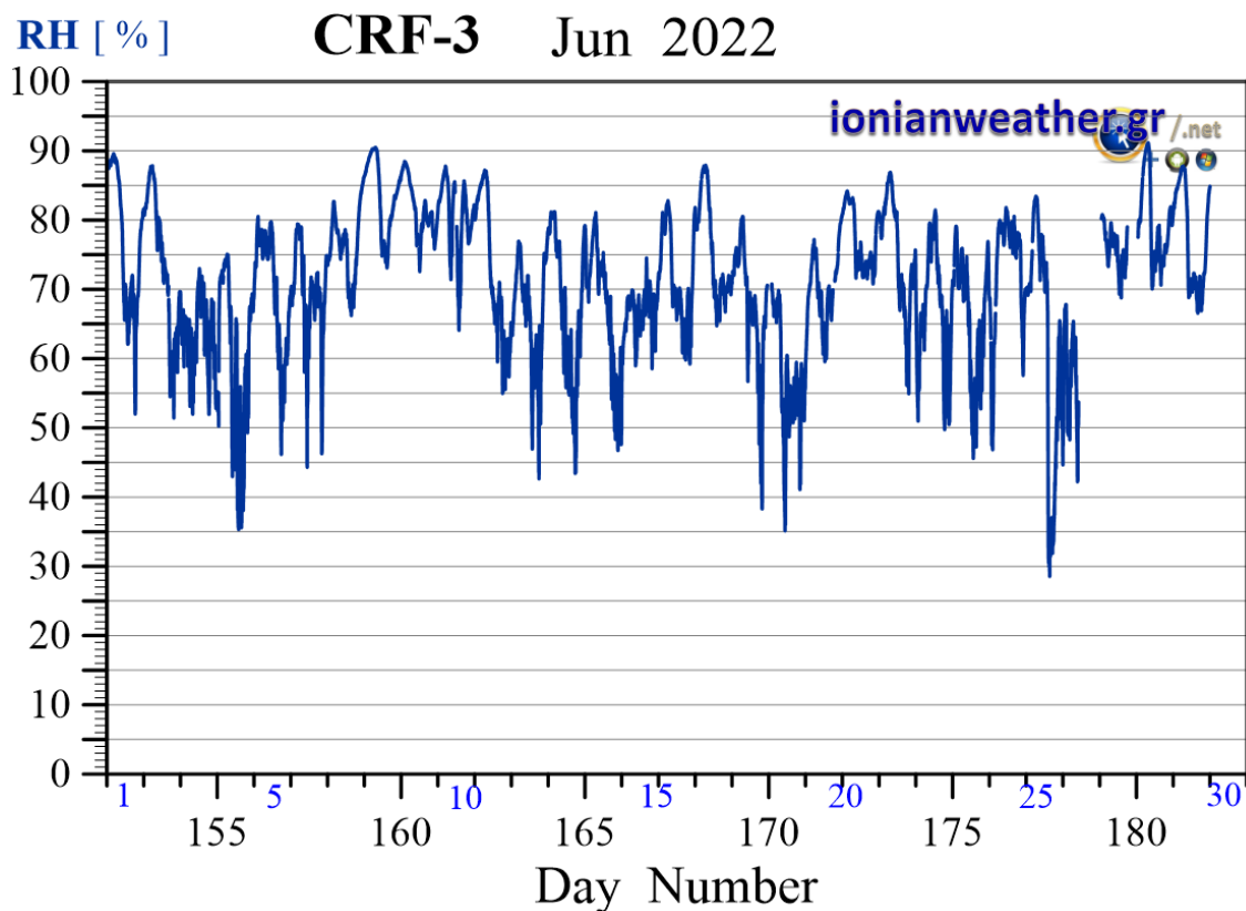
Εικόνα CRF3-5: Μέση ανά λεπτό σχετική υγρασία Ιουνίου 2022.
