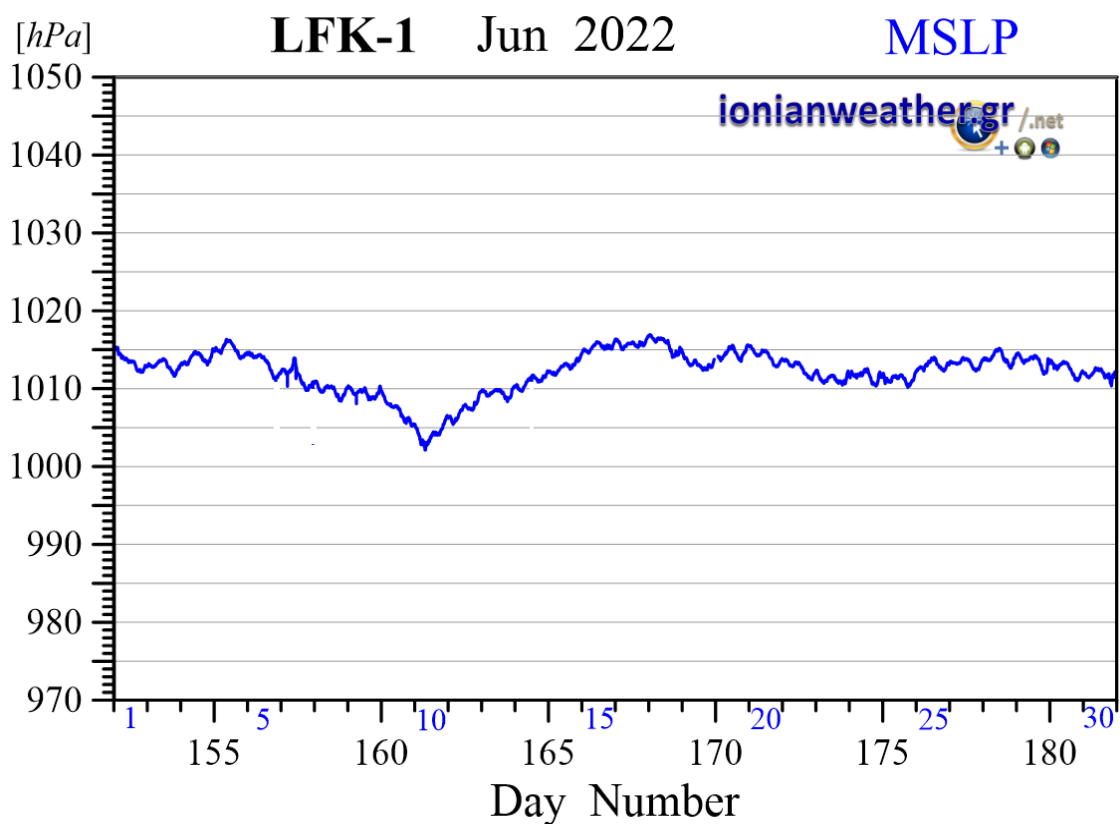
Εικόνα LFK1-6: Μέση ανά λεπτό βαρομετρική πίεση Ιουνίου 2022 ανηγμένη στην επιφάνεια της θάλασσας.
