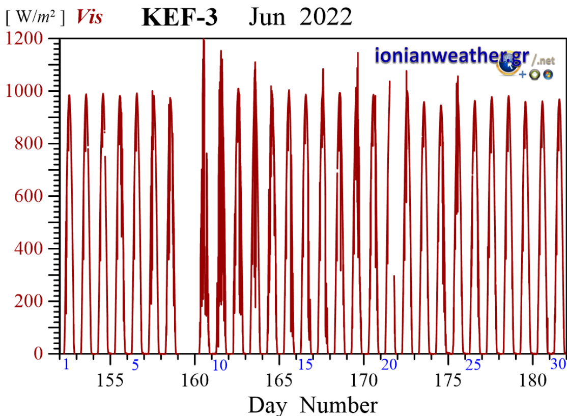
Εικόνα KEF3-7: Μέση ανά λεπτό Ηλιακή ακτινοβολία Ιουνίου 2022 στην οπτική και εγγύς υπέρυθρη περιοχή.
