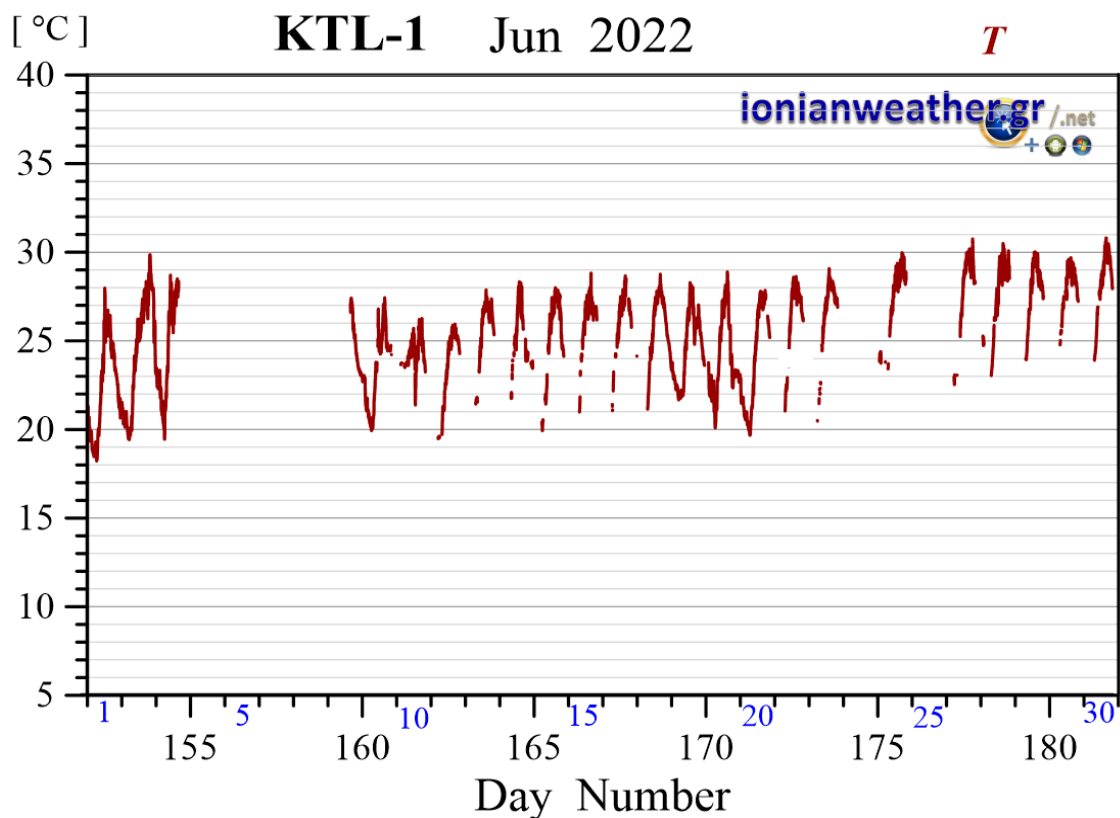
Εικόνα KTL1-4: Μέση ανά λεπτό θερμοκρασία αέρα Ιουνίου 2022.
