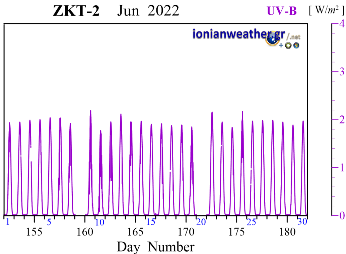
Εικόνα ZKT2-8: Μέση ανά λεπτό Ηλιακή ακτινοβολία Ιουνίου 2022 στην φασματική περιοχή UVB
