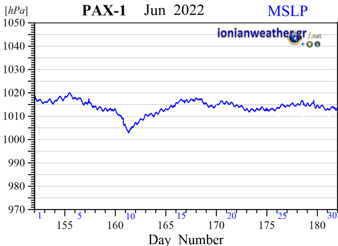
Εικόνα PAX 1-5: Μέση ανά λεπτό βαρομετρική πίεση Ιουνίου 2022 ανηγμένη στην επιφάνεια της θάλασσας.
