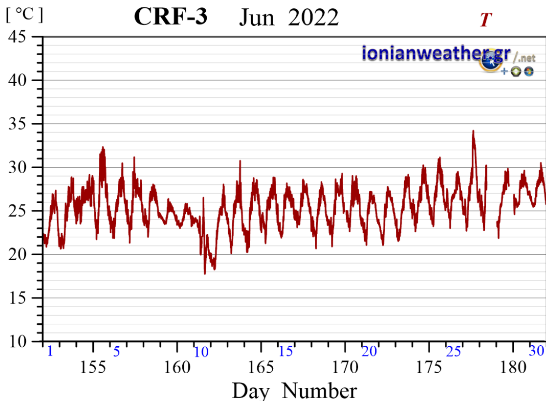
Εικόνα CRF3-4: Μέση ανά λεπτό θερμοκρασία αέρα Ιουνίου 2022.
