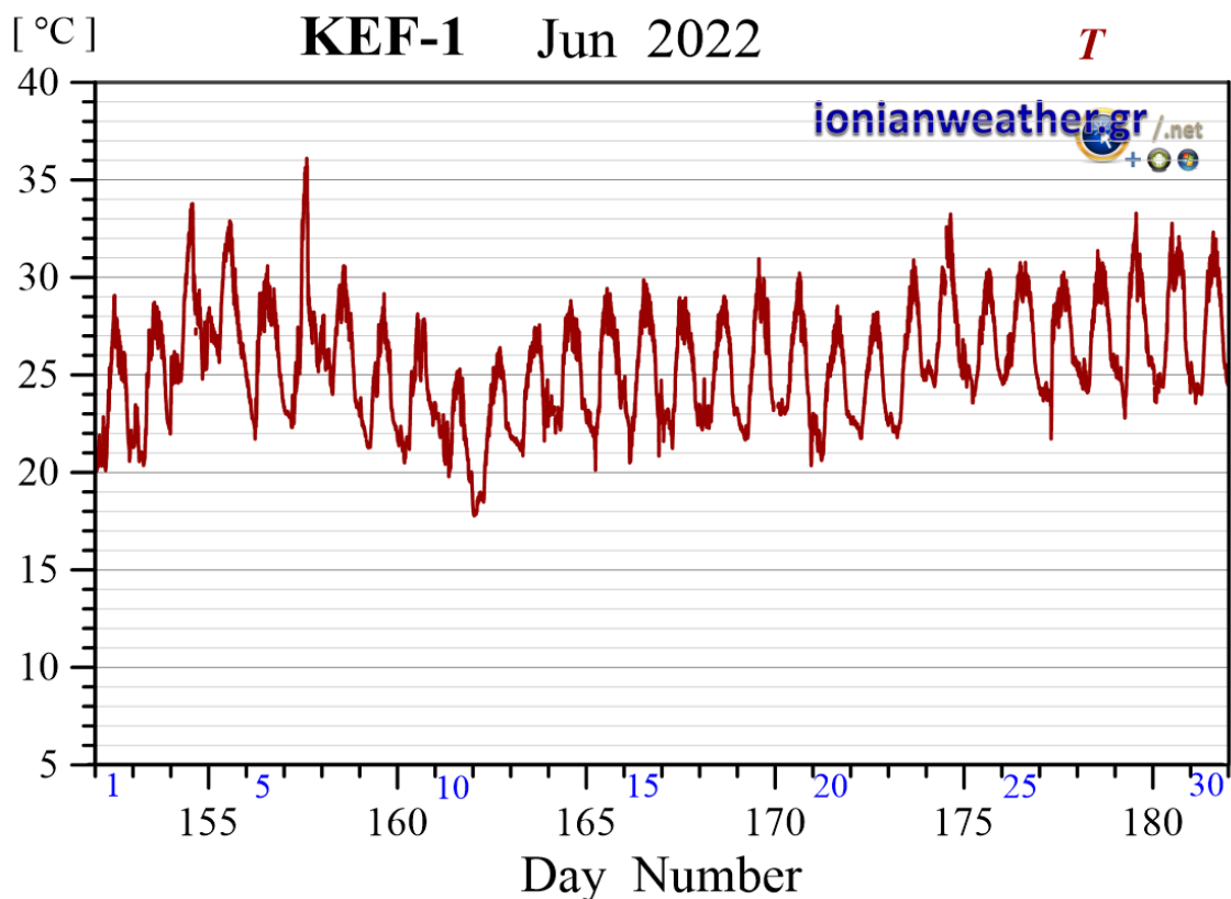
Εικόνα KEF1-4: Μέση ανά λεπτό θερμοκρασία αέρα Ιουνίου 2022.
