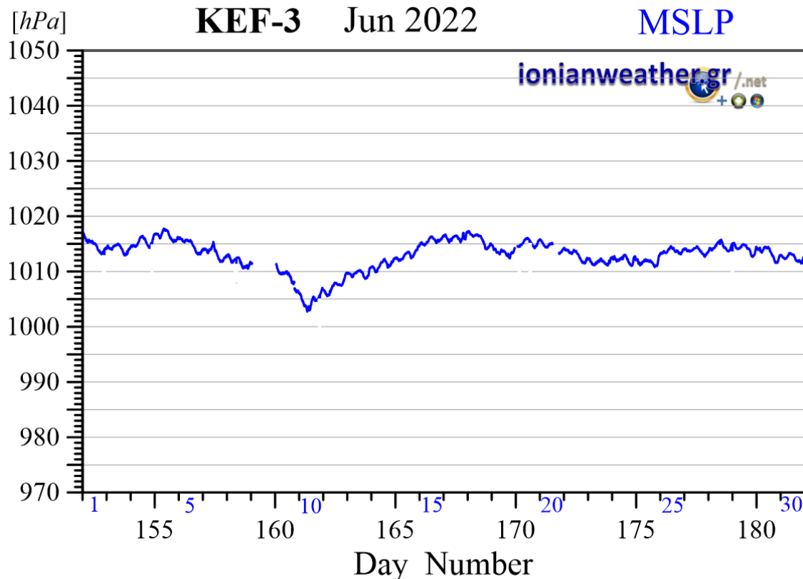
Εικόνα KEF3-6: Μέση ανά λεπτό βαρομετρική πίεση Ιουνίου 2022 ανηγμένη στην επιφάνεια της θάλασσας.
