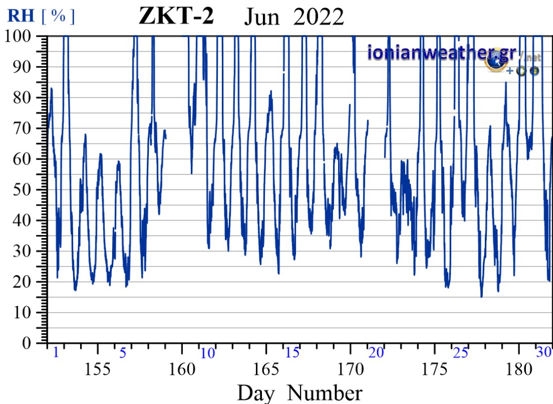
Εικόνα ZKT2-5: Μέση ανά λεπτό σχετική υγρασία Ιουνίου 2022.
