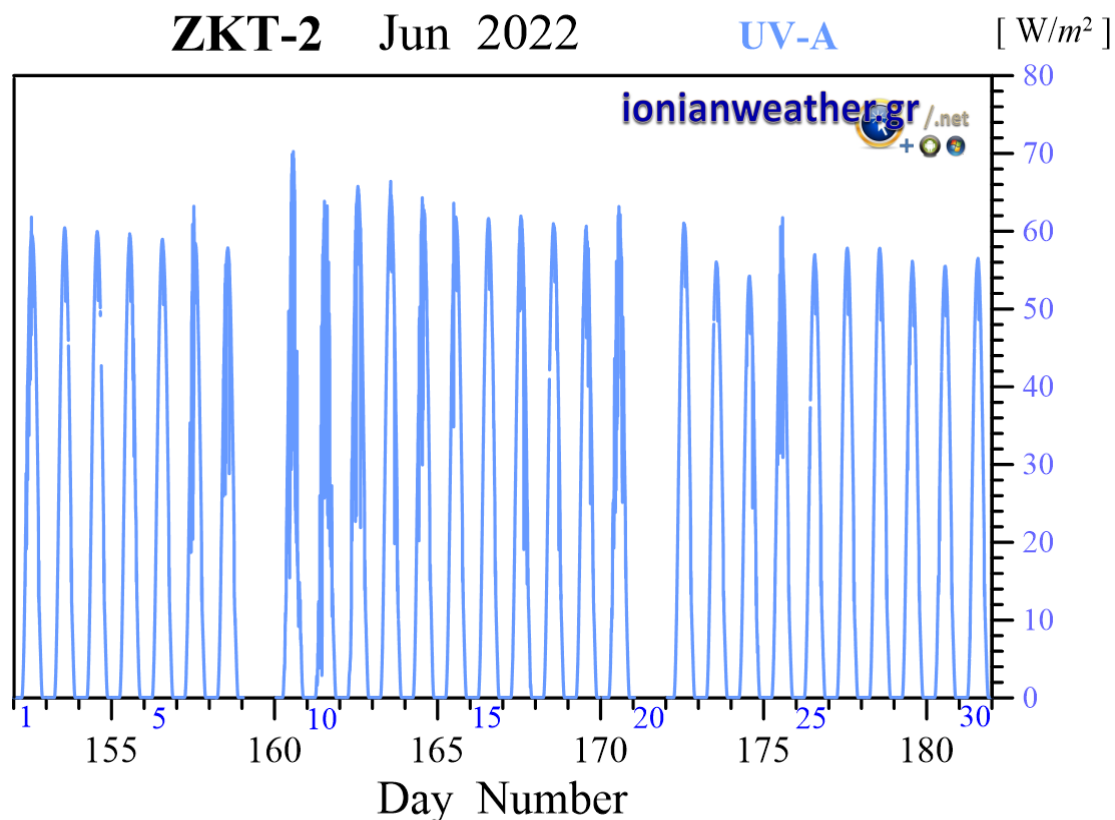
Εικόνα ZKT2-7: Μέση ανά λεπτό Ηλιακή ακτινοβολία Ιουνίου 2022 στη φασματική περιοχή UVA.
