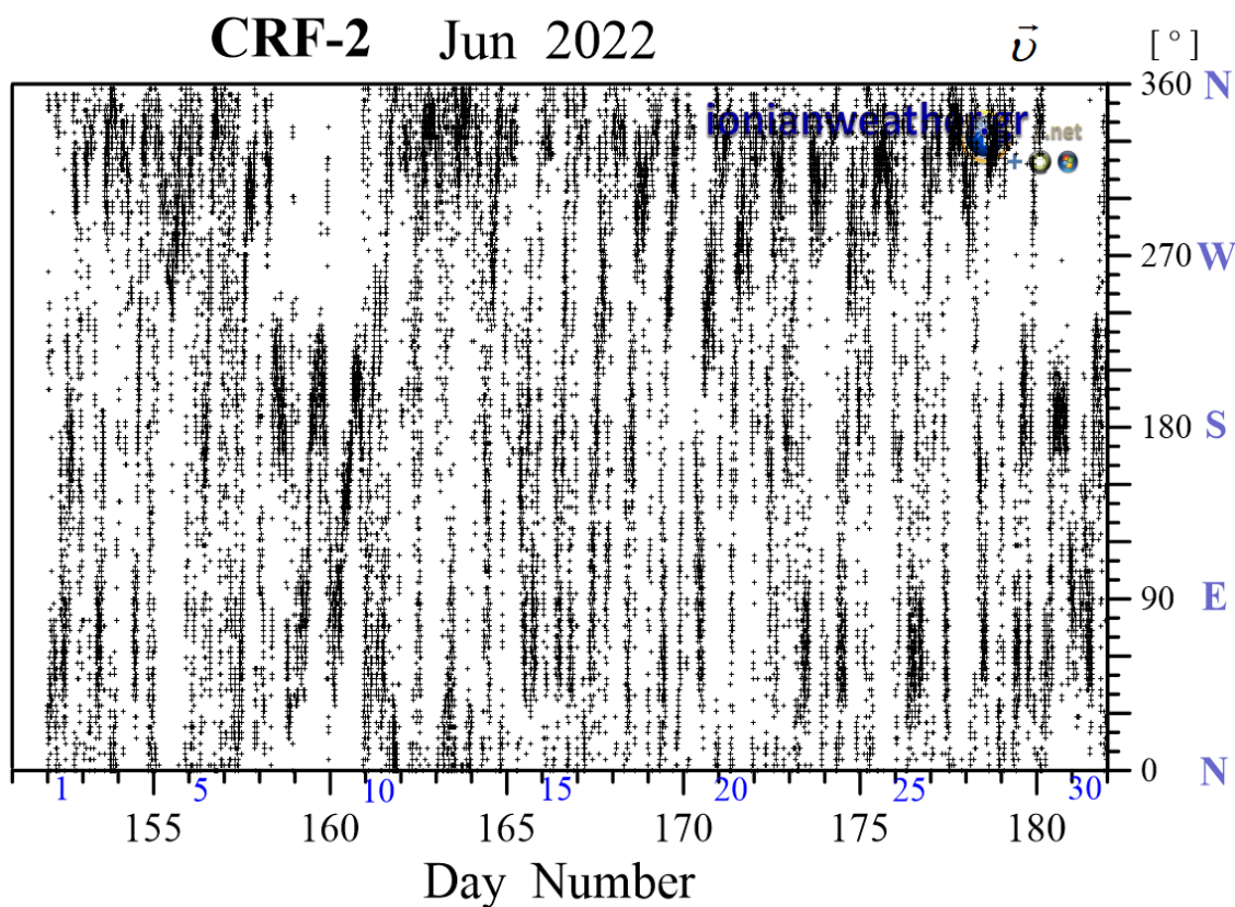
Εικόνα CRF2-3: Μέση ανά λεπτό κατεύθυνση ανέμου Ιουνίου 2022 (κλίμακα αζιμουθίων δεξιά)
