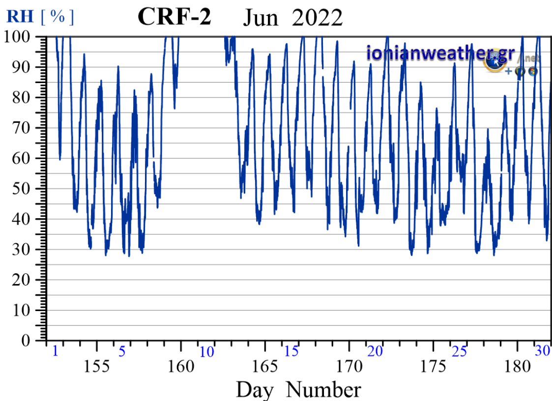
Εικόνα CRF2-5: Μέση ανά λεπτό σχετική υγρασία Ιουνίου 2022.
