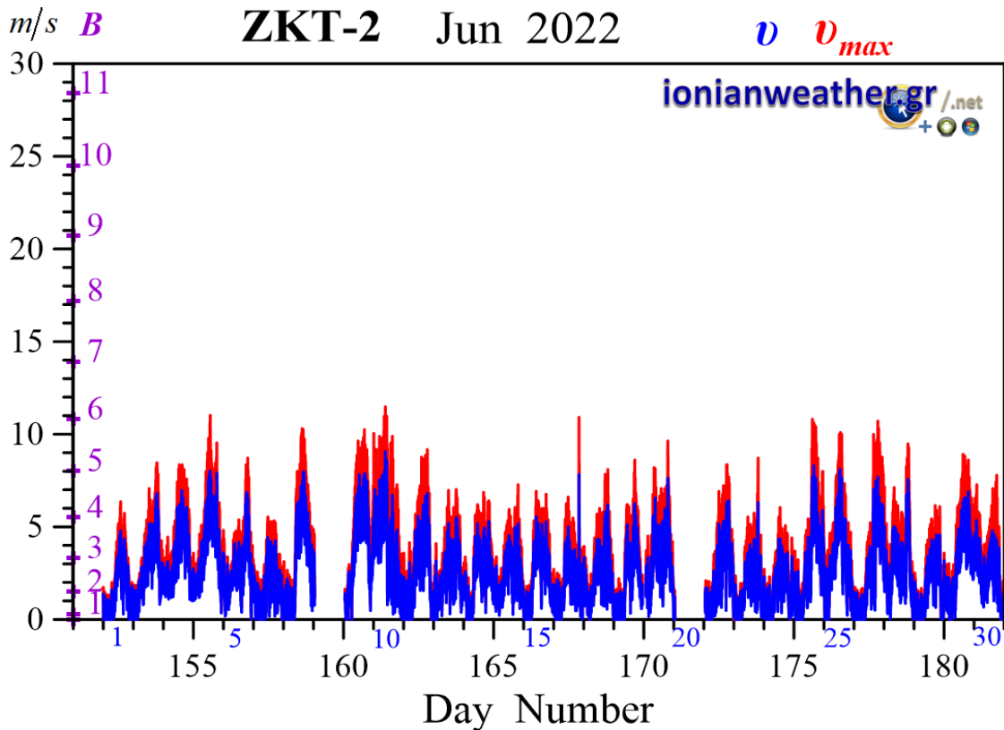
Εικόνα ZKT2-2: Μέση ανά λεπτό ταχύτητα ανέμου (m/s, γαλάζιο) και ριπή ανέμου (κόκκινο) Ιουνίου 2022. Κλίμακα ταχυτήτων αριστερά σε m/s και Beaufort.
