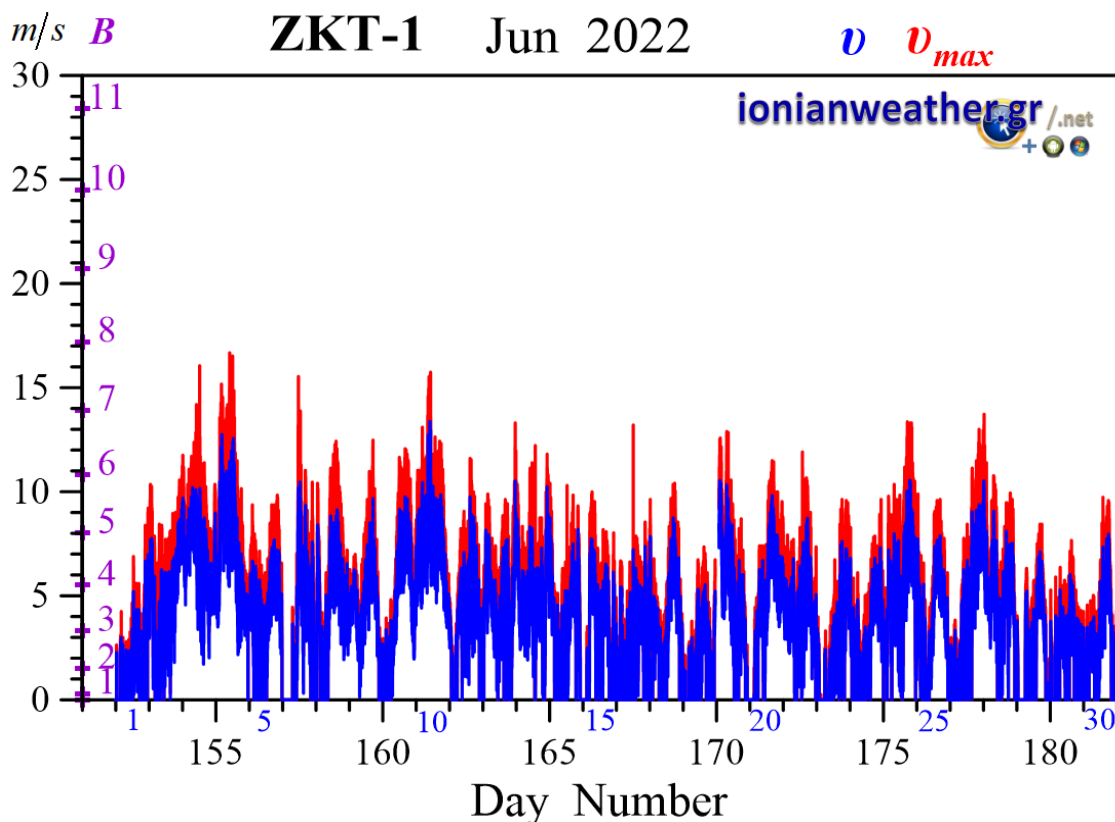
Εικόνα ZKT1-2: Μέση ανά λεπτό ταχύτητα ανέμου ( m/s , γαλάζιο) και ριπή ανέμου (κόκκινο) Ιουνίου 2022. Κλίμακα ταχυτήτων αριστερά σε m/s και Beaufort .
