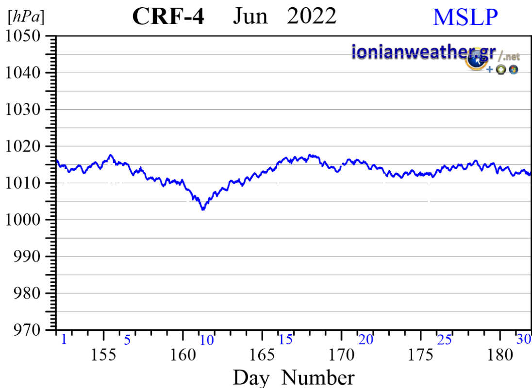
Εικόνα CRF4-6: Μέση ανά λεπτό βαρομετρική πίεση Ιουνίου 2022 ανηγμένη στην επιφάνεια της θάλασσας.
