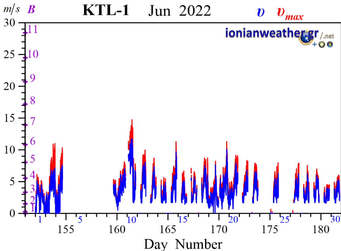
Εικόνα KTL1-2: Μέση ανά λεπτό ταχύτητα ανέμου ( m/s , γαλάζιο) και ριπή ανέμου (κόκκινο) Ιουνίου 2022. Κλίμακα ταχυτήτων αριστερά σε m/s και Beaufort.
