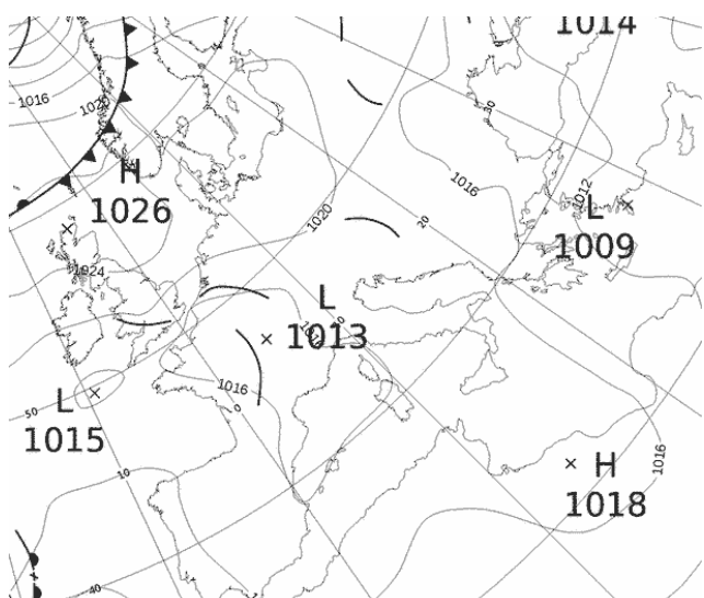
Εικόνα 3.1-5: MSLP 5 June 2022 00UTC
