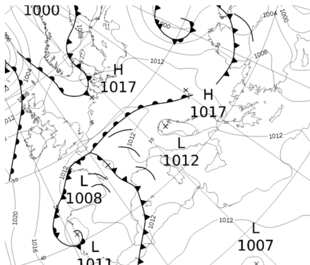
Εικόνα 3.1-22: MSLP 22 June 2022 00UTC
