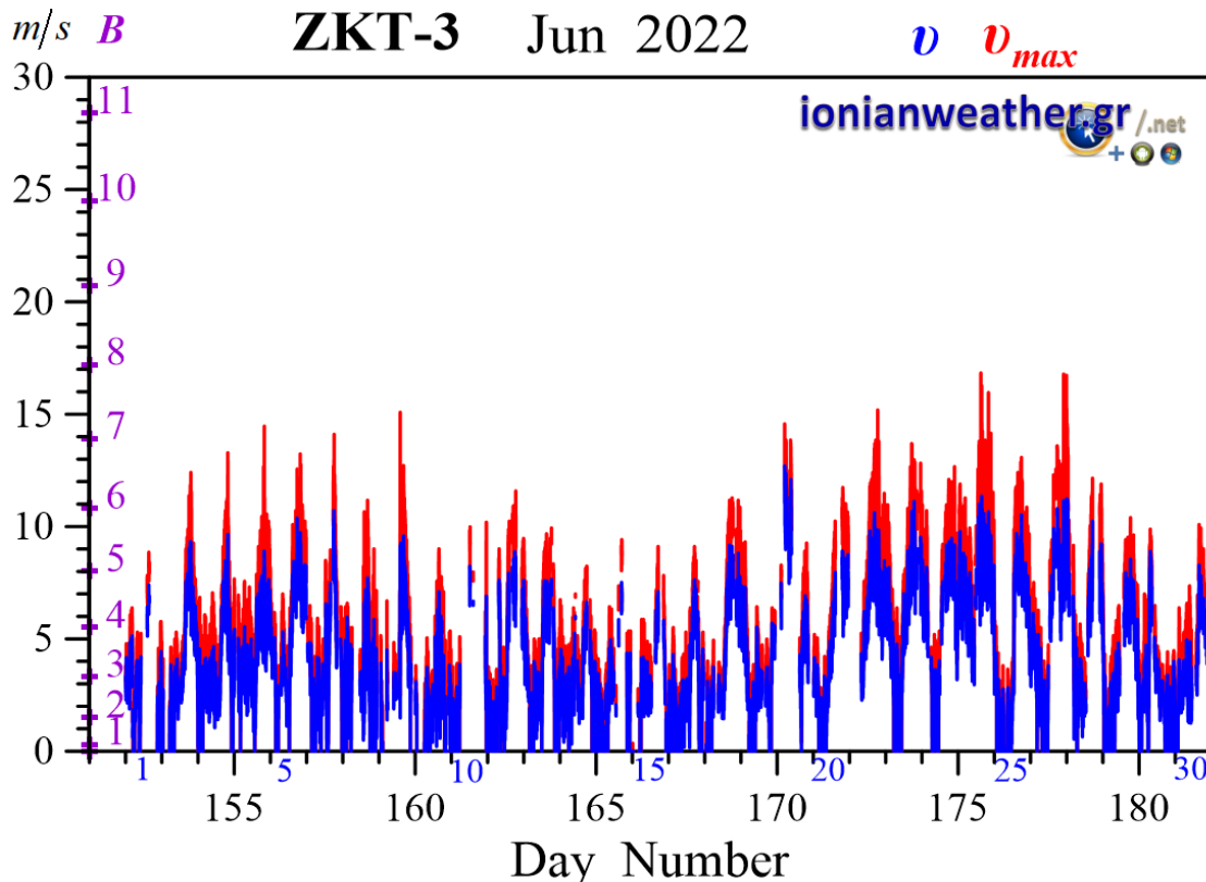
Εικόνα ZKT3-2: Μέση ανά λεπτό ταχύτητα ανέμου (m/s, γαλάζιο) και ριπή ανέμου (κόκκινο) Ιουνίου 2022. Κλίμακα ταχυτήτων αριστερά σε m/s και Beaufort.
