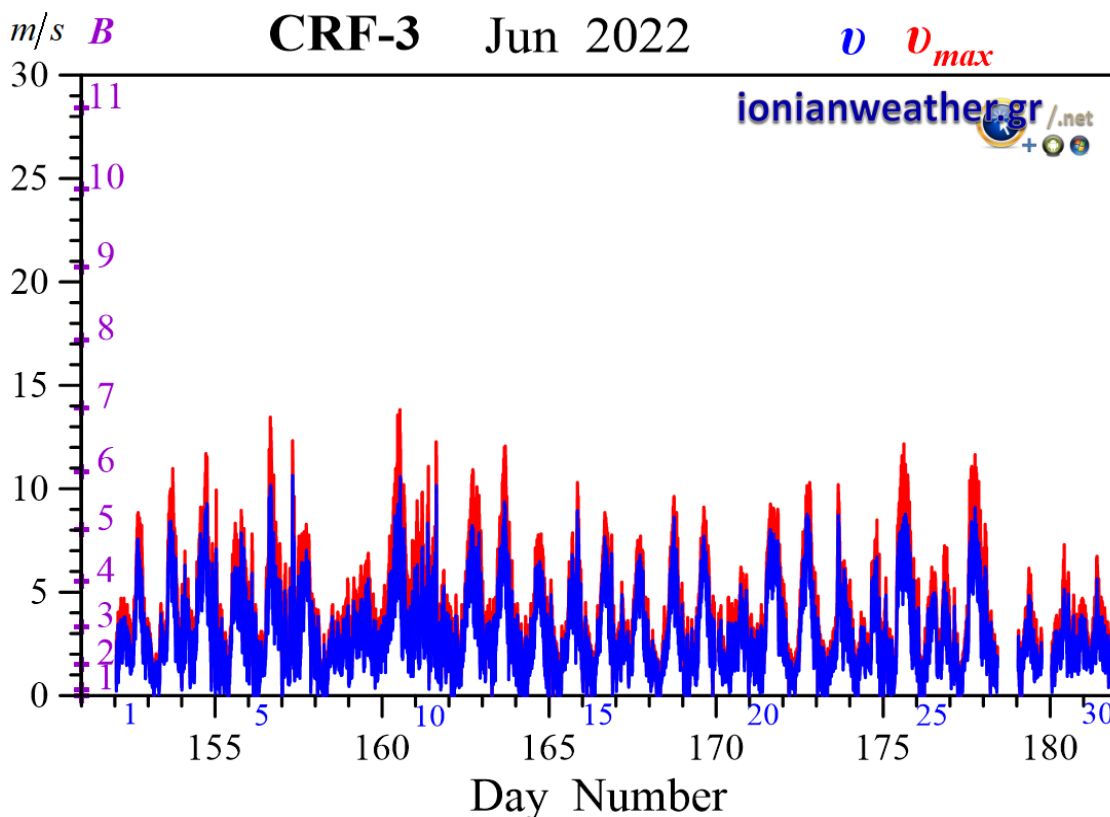
Εικόνα CRF3-2: Μέση ανά λεπτό ταχύτητα ανέμου (m/s, γαλάζιο) και ριπή ανέμου (κόκκινο) Ιουνίου 2022. Κλίμακα ταχυτήτων αριστερά σε m/s και Beaufort.
