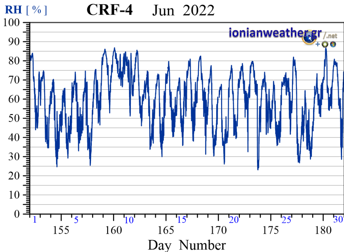
Εικόνα CRF4-5: Μέση ανά λεπτό σχετική υγρασία Ιουνίου 2022.
