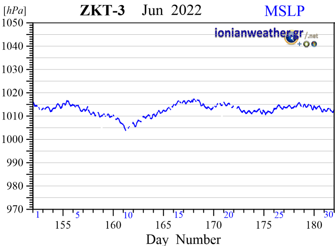
Εικόνα ZKT3-6: Μέση ανά λεπτό βαρομετρική πίεση Ιουνίου 2022 ανηγμένη στην επιφάνεια της θάλασσας.
