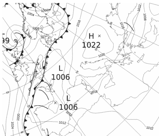
Εικόνα 3.1-19: MSLP 19 June 2022 00UTC
