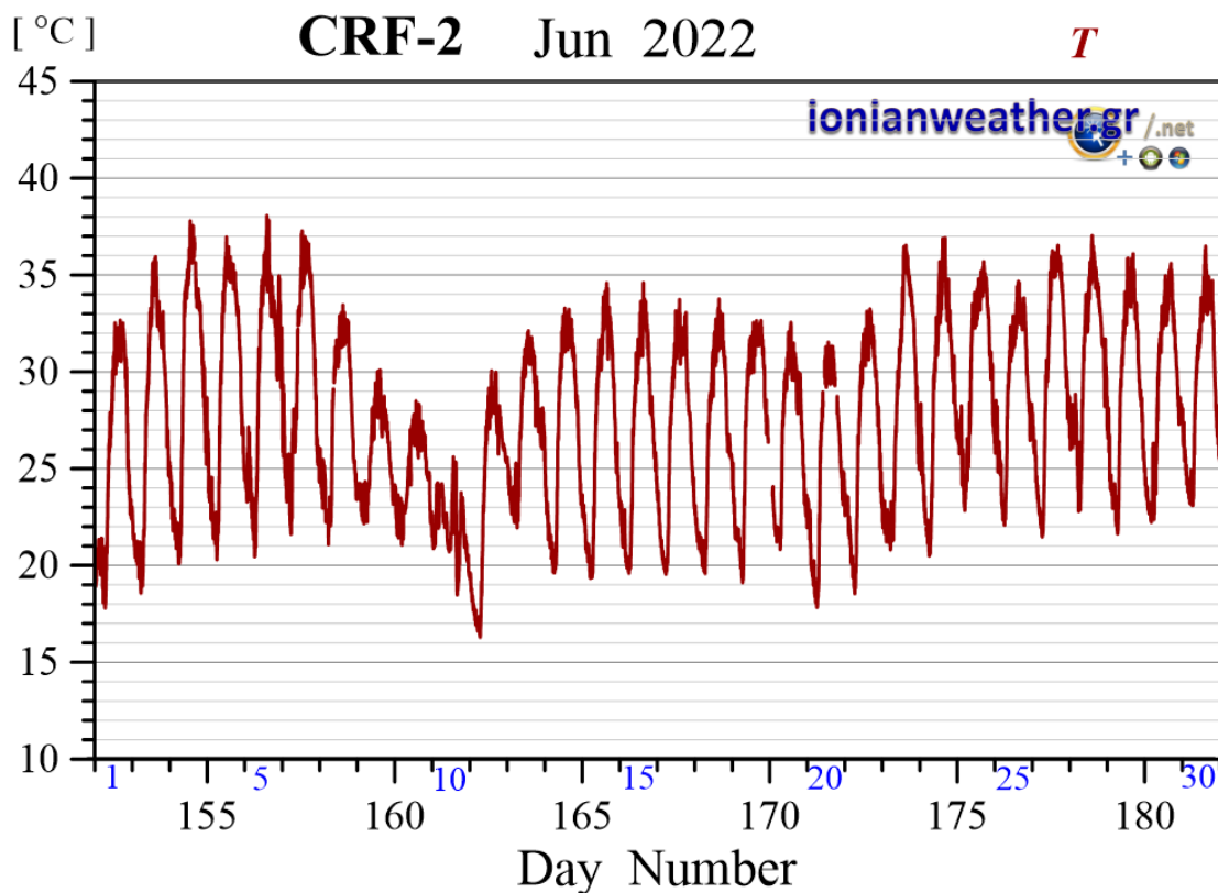
Εικόνα CRF2-4: Μέση ανά λεπτό θερμοκρασία αέρα Ιουνίου 2022.
