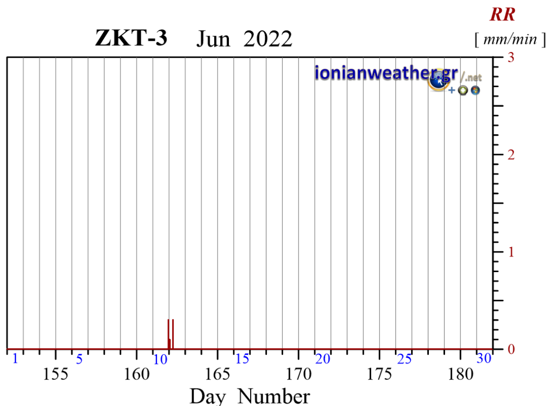
Εικόνα ZKT3-1: Ανά λεπτό ρυθμός βροχόπτωσης (mm/min) Ιουνίου 2022.
