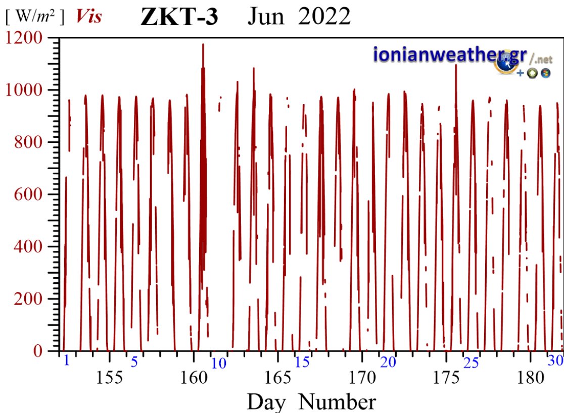
Εικόνα ZKT3-7: Μέση ανά λεπτό Ηλιακή ακτινοβολία Ιουνίου 2022 στην οπτική και εγγύς υπέρυθρη περιοχή.
