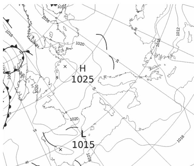
Εικόνα 3.1-17: MSLP 17 June 2022 00UTC
