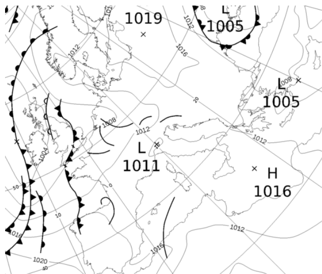
Εικόνα 3.1-24: MSLP 24 June 2022 00UTC
