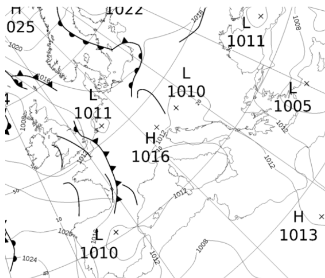
Εικόνα 3.1-30: MSLP 30 June 2022 00UTC
