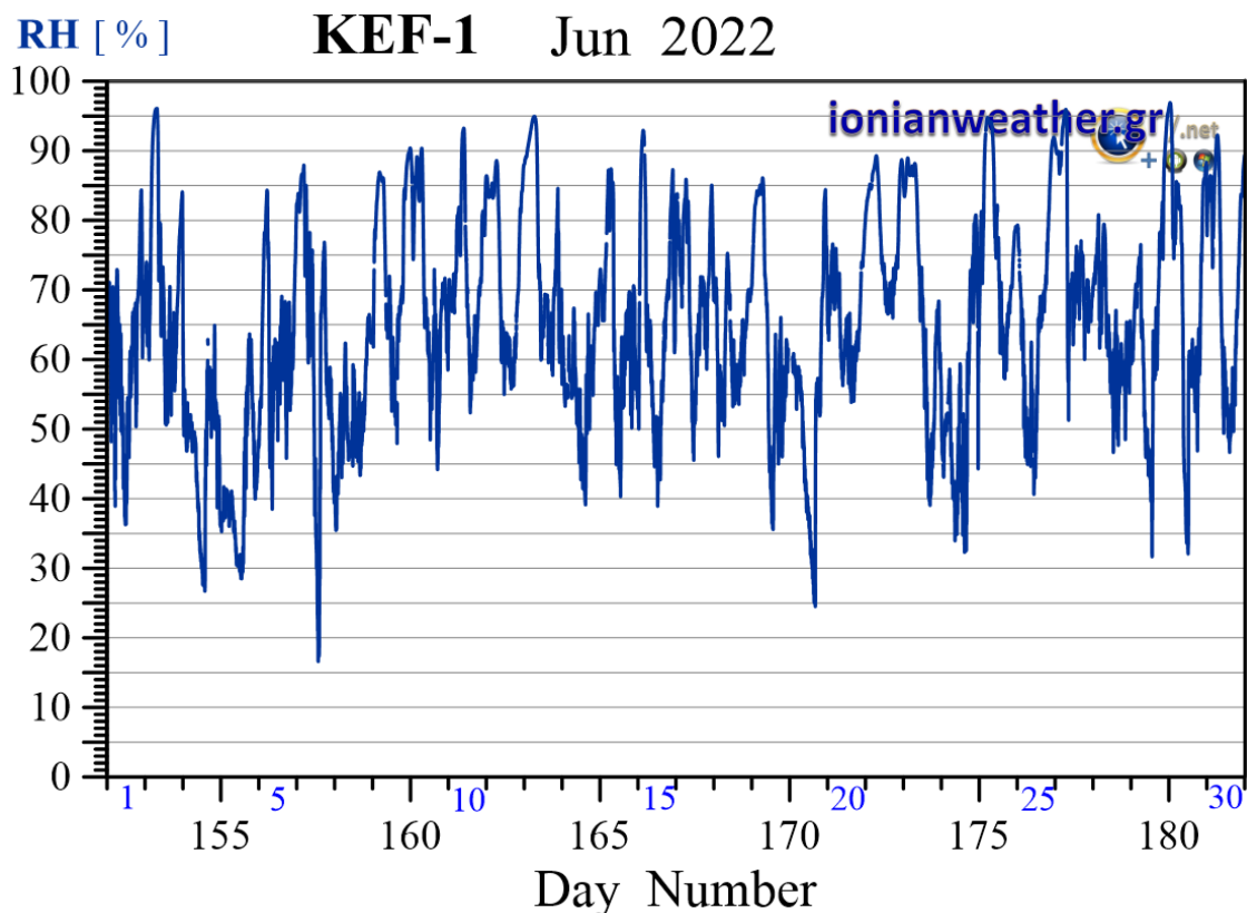
Εικόνα KEF1-5: Μέση ανά λεπτό σχετική υγρασία Ιουνίου 2022.
