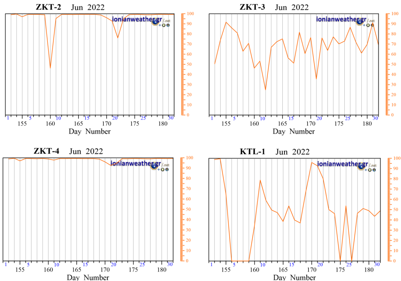
Εικόνα 2.3: Ημερήσιες τιμές πληρότητας ροής δεδομένων μέσω του δικτύου GSM και της υπηρεσίας GPRS απο τους Μετεωρολογικούς σταθμούς προς τον κεντρικό server, για τον Ιούνιο 2022 (κλίμακα ημερήσιας πληρότητας σε %, στα δεξιά).
