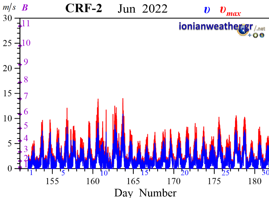
Εικόνα CRF2-2: Μέση ανά λεπτό ταχύτητα ανέμου ( m/s , γαλάζιο) και ριπή ανέμου (κόκκινο) Ιουνίου 2022. Κλίμακα ταχυτήτων αριστερά σε m/s και Beaufort .
