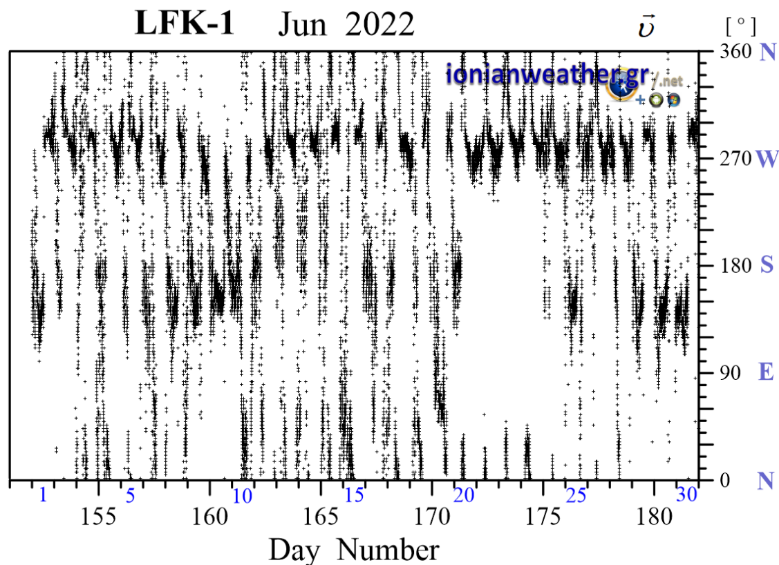
Εικόνα LFK1-3: Μέση ανά λεπτό κατεύθυνση ανέμου Ιουνίου 2022 (κλίμακα αζιμουθίων δεξιά)
