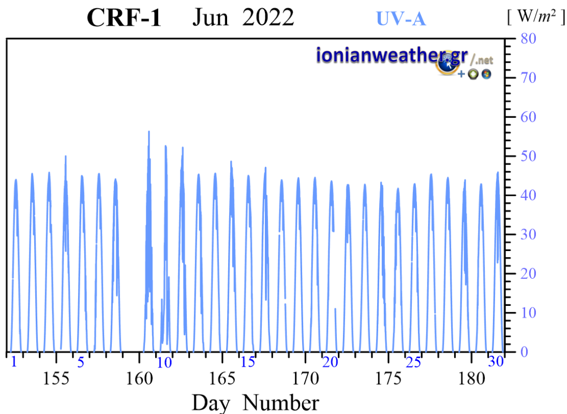
Εικόνα CRF1-8: Μέση ανά λεπτό Ηλιακή ακτινοβολία Ιουνίου 2022 στη φασματική περιοχή UVA.
