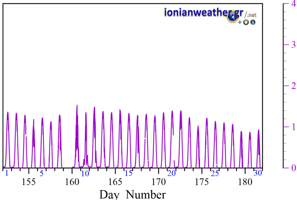
Εικόνα CRF1-9: Μέση ανά λεπτό Ηλιακή ακτινοβολία Ιουνίου 2022 στη φασματική περιοχή UVB.
