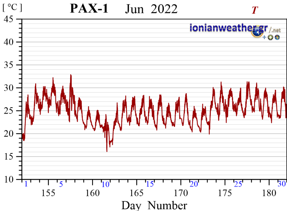
Εικόνα PAX 1-4: Μέση ανά λεπτό θερμοκρασία αέρα Ιουνίου 2022.
