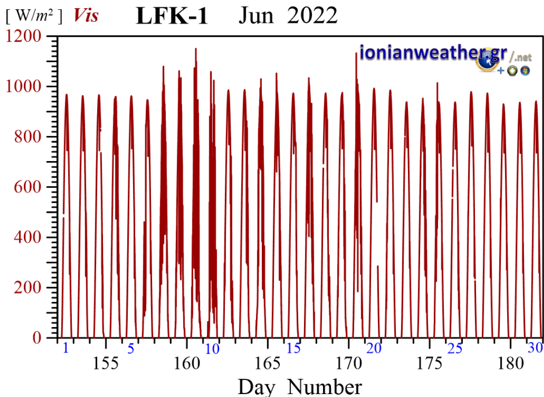
Εικόνα LFK1-7: Μέση ανά λεπτό Ηλιακή ακτινοβολία Ιουνίου 2022 στην οπτική και εγγύς υπέρυθρη περιοχή.
