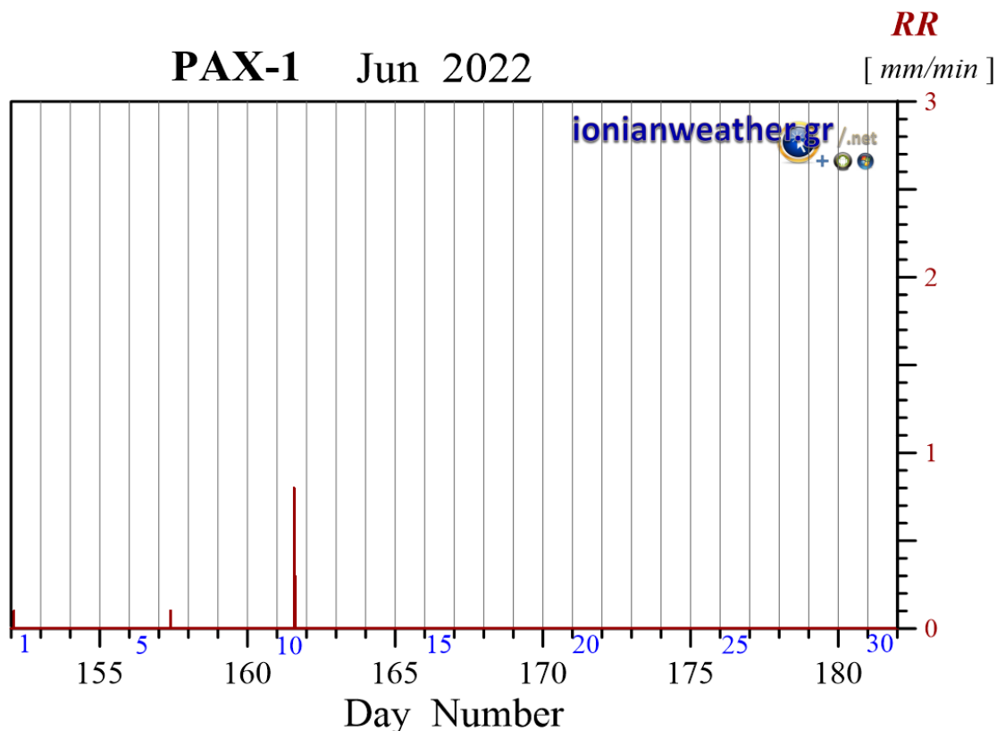
Εικόνα PAX1-1: Ανά λεπτό ρυθμός βροχόπτωσης (mm/min) Ιουνίου 2022.
