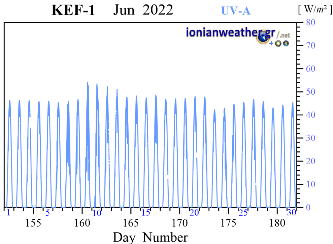
Εικόνα KEF1-8: Μέση ανά λεπτό Ηλιακή ακτινοβολία Ιουνίου 2022 στη φασματική περιοχή UVA.
