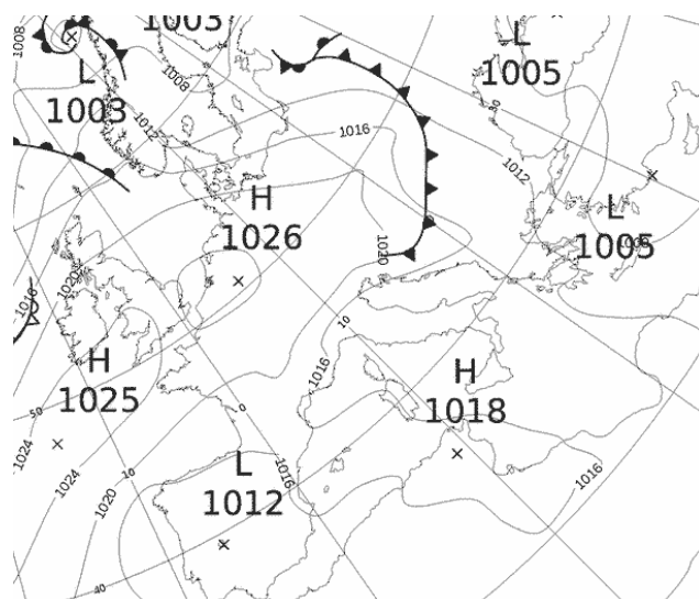
Εικόνα 3.1-14: MSLP 14 June 2022 00UTC
