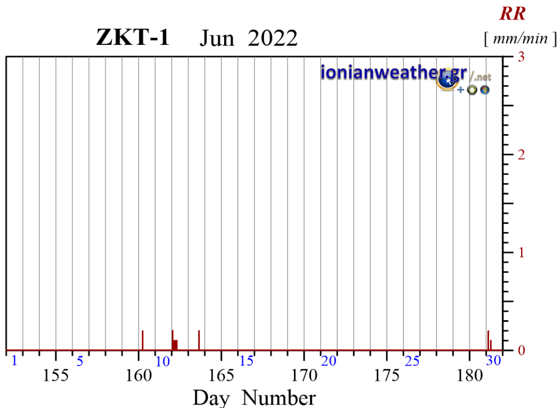
Εικόνα ZKT1-1: Ανά λεπτό ρυθμός βροχόπτωσης (mm/min) Ιουνίου 2022.
