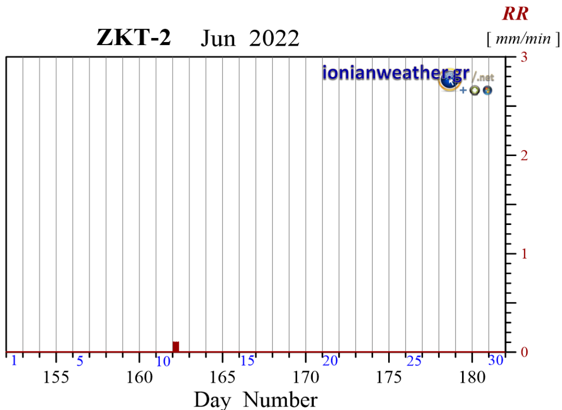
Εικόνα ZKT2-1: Ανά λεπτό ρυθμός βροχόπτωσης (mm/min) Ιουνίου 2022.
