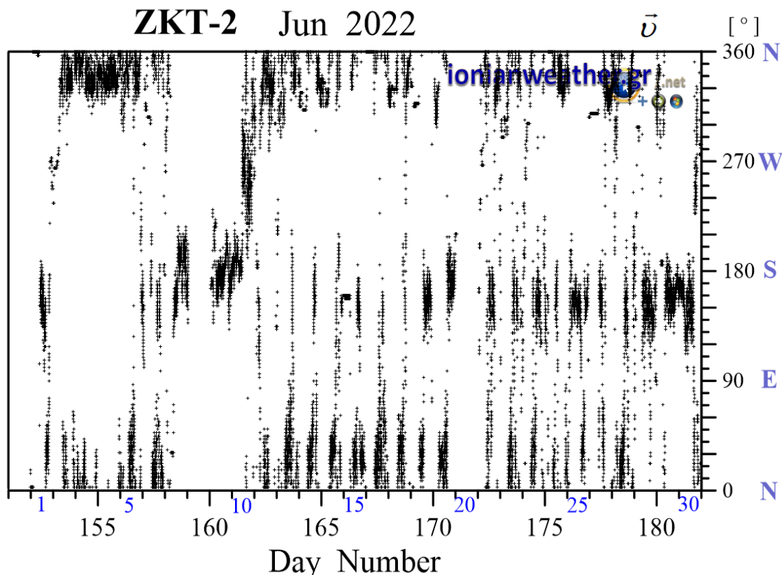
Εικόνα ZKT2-3: Μέση ανά λεπτό κατεύθυνση ανέμου Ιουνίου 2022 (κλίμακα αζιμουθίων δεξιά)
