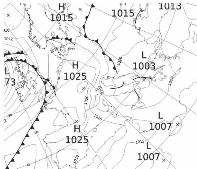
Εικόνα 3.1-10: MSLP 10 June 2022 00UTC
