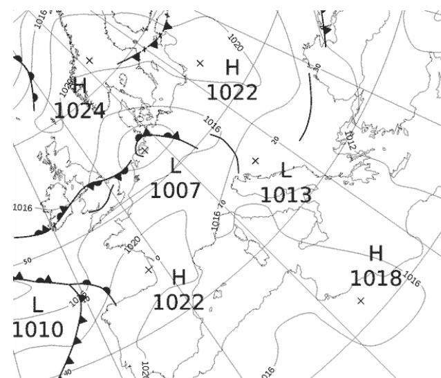
Εικόνα 3.1-6: MSLP 6 June 2022 00UTC
