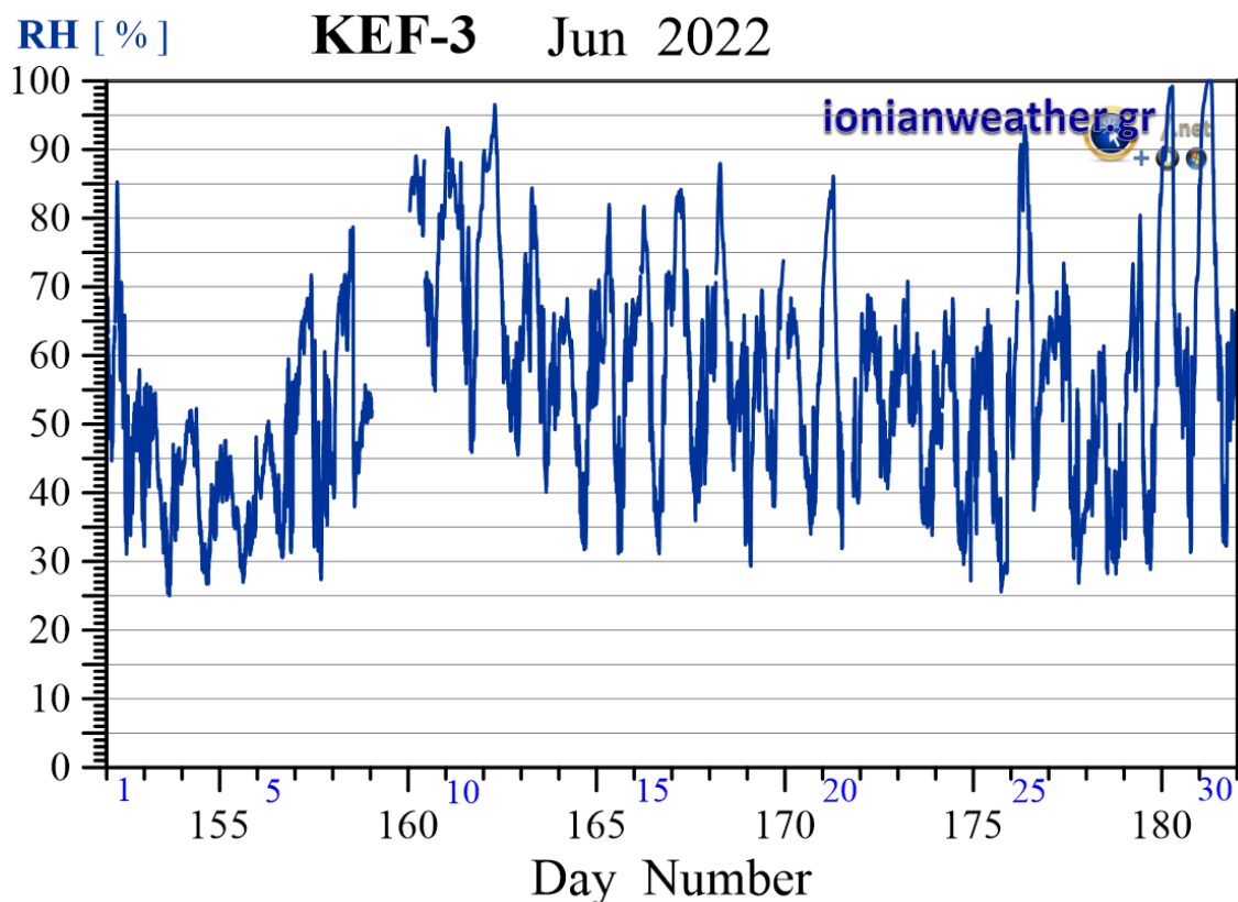
Εικόνα KEF3-5: Μέση ανά λεπτό σχετική υγρασία Ιουνίου 2022.
