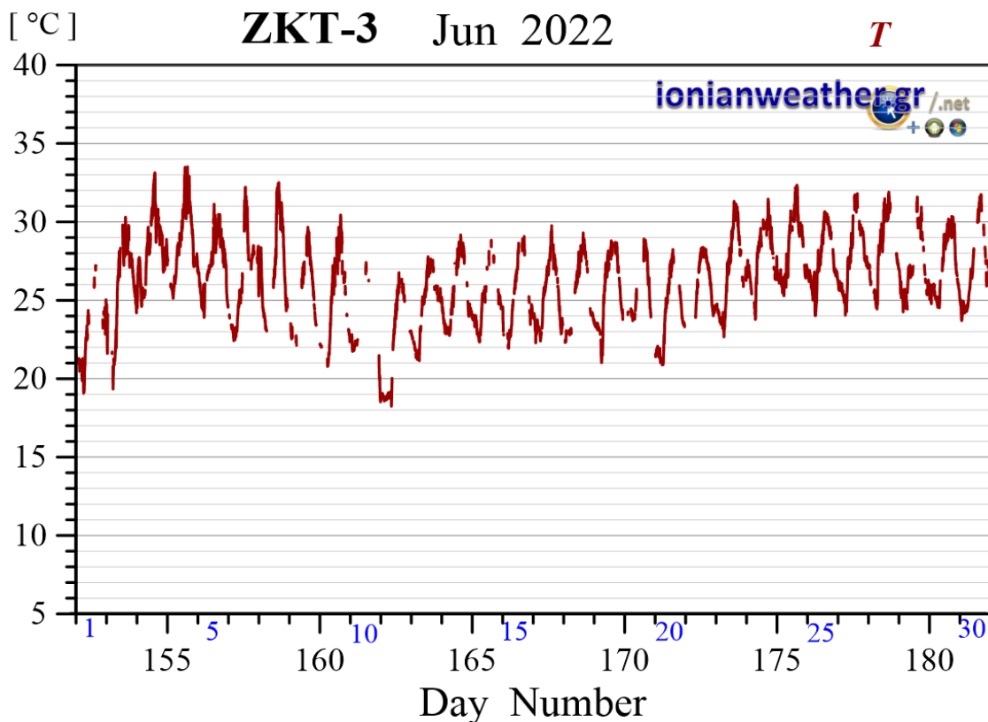
Εικόνα ZKT3-4: Μέση ανά λεπτό θερμοκρασία αέρα Ιουνίου 2022.
