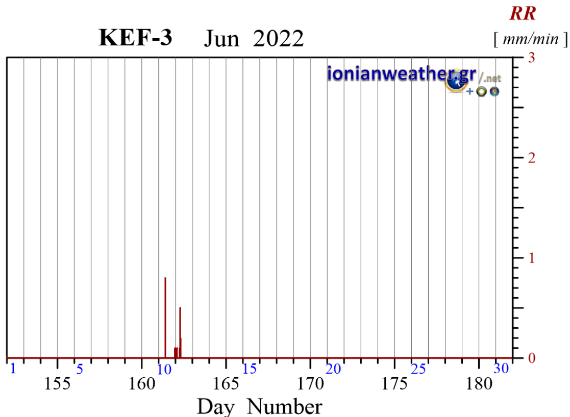
Εικόνα KEF3-1: Ανά λεπτό ρυθμός βροχόπτωσης ( mm/min ) Ιουνίου 2022.
