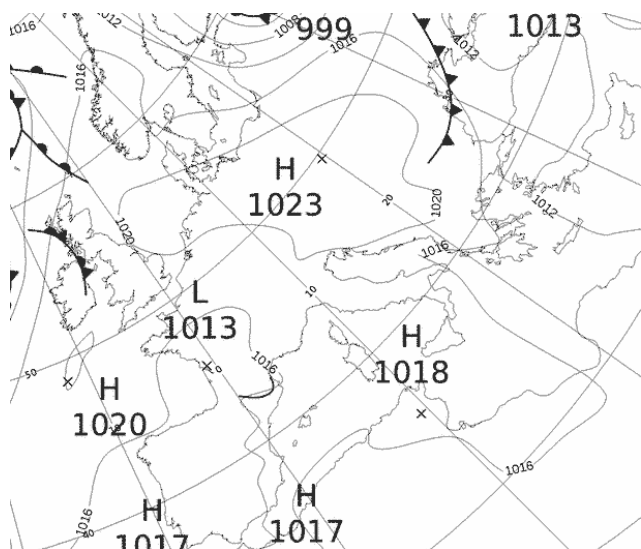
Εικόνα 3.1-15: MSLP 15 June 2022 00UTC
