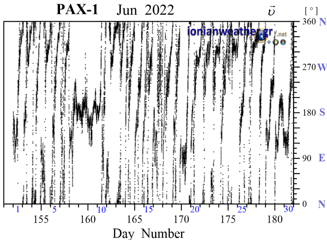
Εικόνα PAX 1-3: Μέση ανά λεπτό κατεύθυνση ανέμου Ιουνίου 2022 (κλίμακα αζιμουθίων δεξιά)
