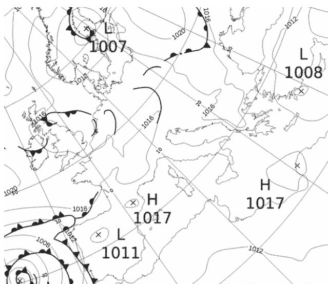
Εικόνα 3.1-1: MSLP 1 June 2022 00UTC
