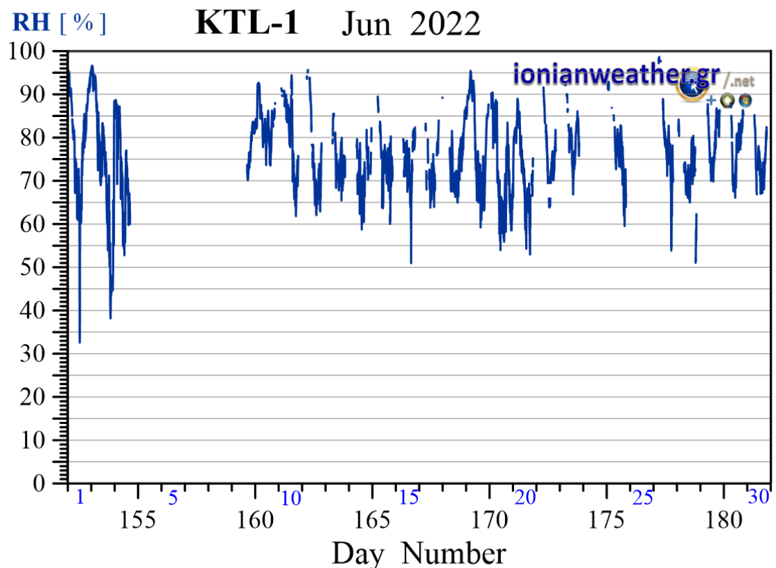
Εικόνα KTL1-5: Μέση ανά λεπτό σχετική υγρασία Ιουνίου 2022.
