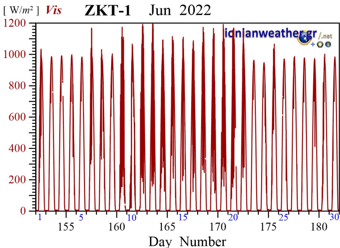
Εικόνα ZKT1-7: Μέση ανά λεπτό Ηλιακή ακτινοβολία Ιουνίου 2022 στην οπτική και εγγύς υπέρυθρη περιοχή.
