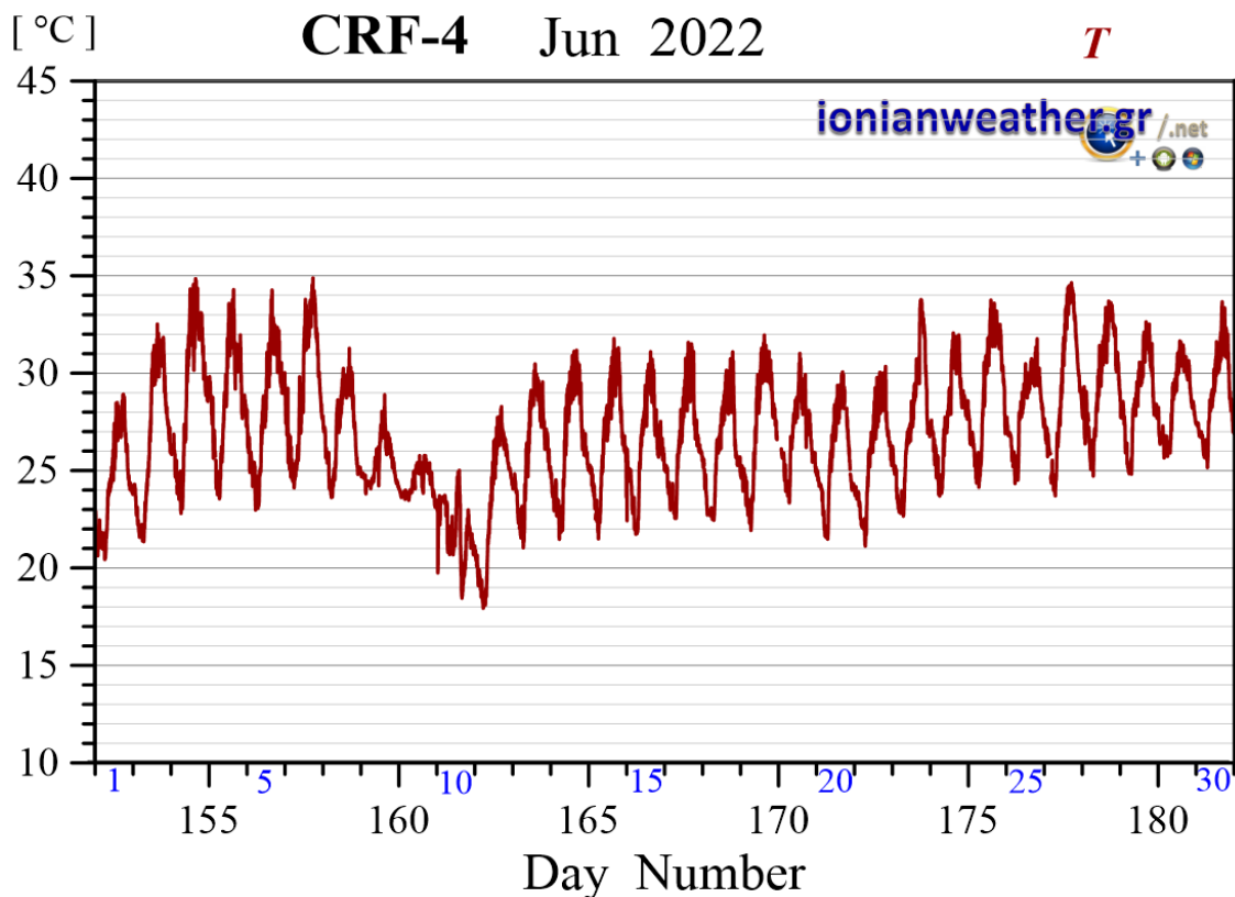
Εικόνα CRF4-4: Μέση ανά λεπτό θερμοκρασία αέρα Ιουνίου 2022.
