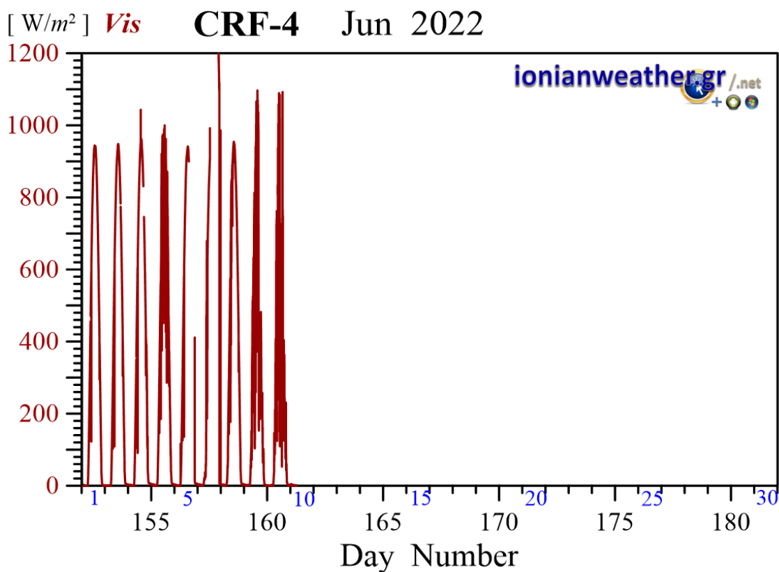
Εικόνα CRF4-7: Μέση ανά λεπτό Ηλιακή ακτινοβολία Ιουνίου 2022 στην οπτική και εγγύς υπέρυθρη περιοχή.
