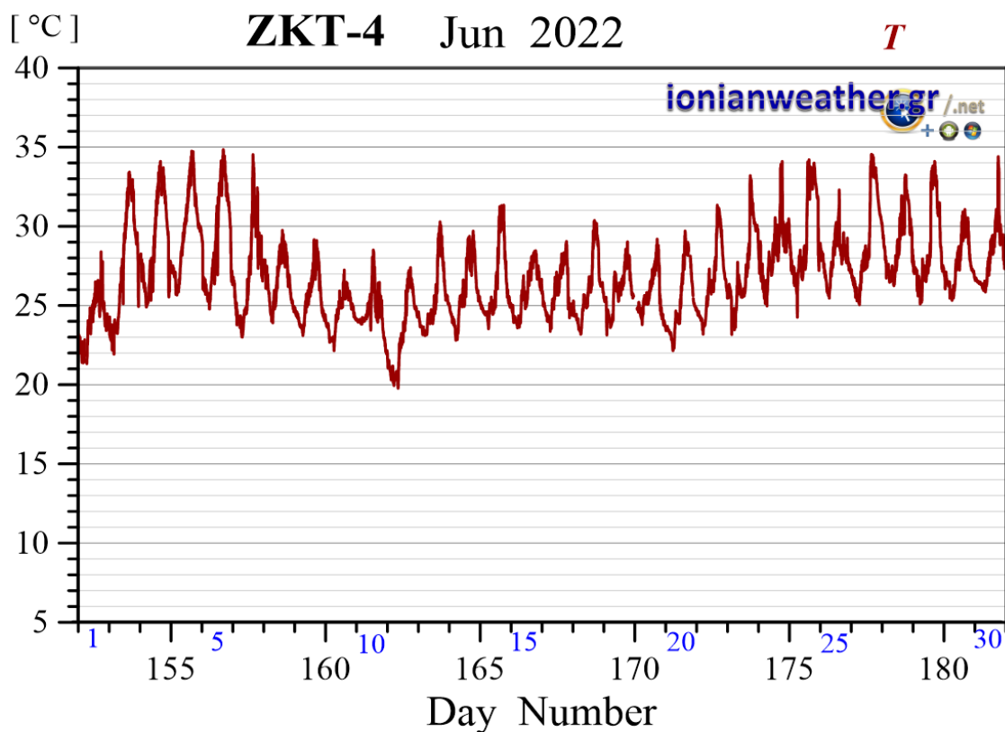
Εικόνα ZKT4-4: Μέση ανά λεπτό θερμοκρασία αέρα Ιουνίου 2022.
