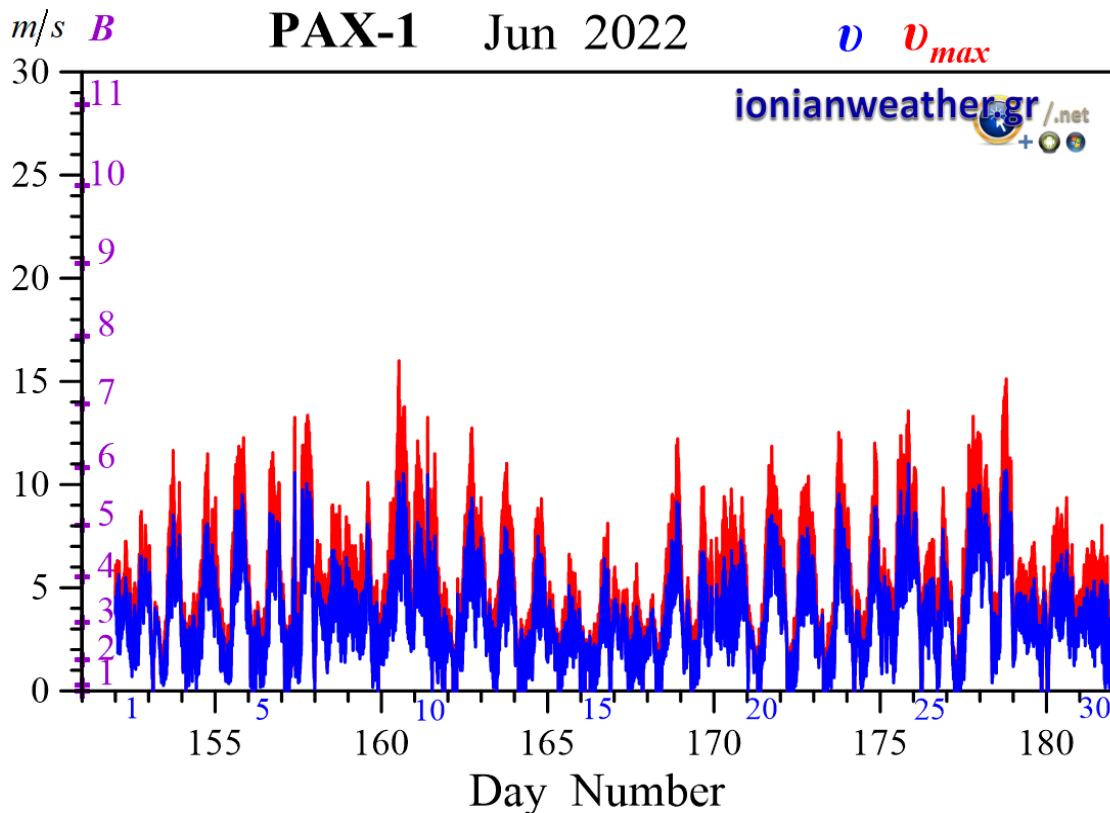
Εικόνα PAX 1-2: Μέση ανά λεπτό ταχύτητα ανέμου (m/s, γαλάζιο) και ριπή ανέμου (κόκκινο) Ιουνίου 2022. Κλίμακα ταχυτήτων αριστερά σε m/s και Beaufort.
