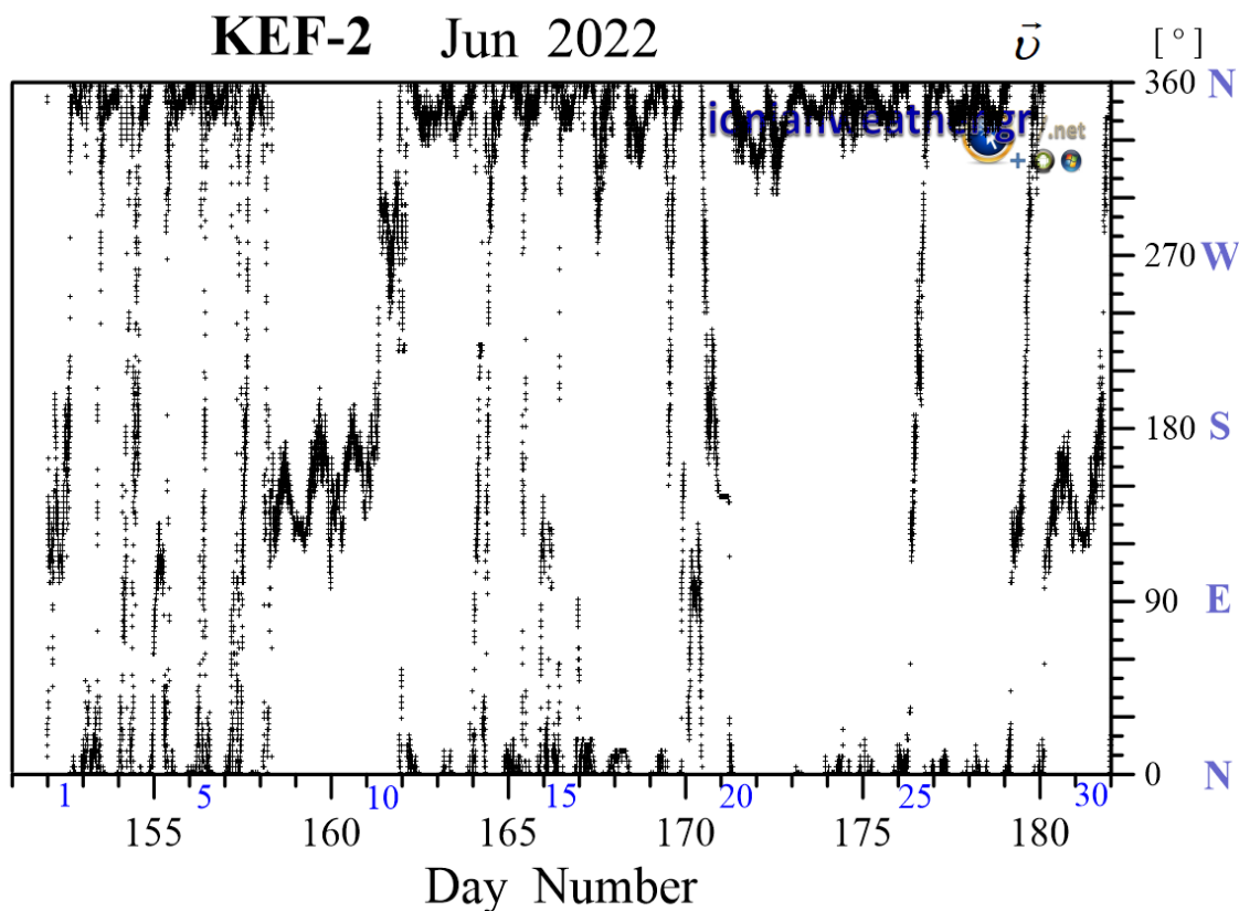
Εικόνα KEF2-3: Μέση ανά λεπτό κατεύθυνση ανέμου Ιουνίου 2022 (κλίμακα αζιμουθίων δεξιά)
