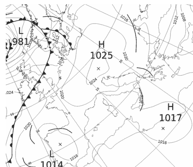
Εικόνα 3.1-18: MSLP 18 June 2022 00UTC
