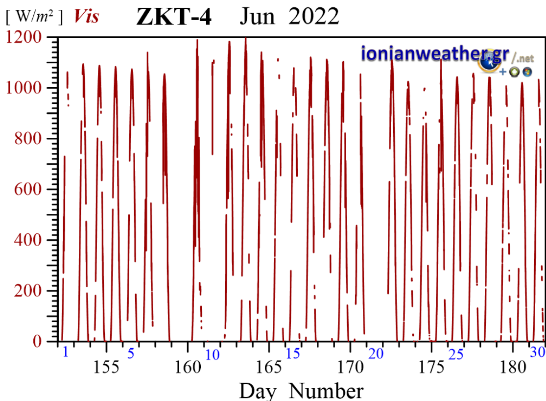
Εικόνα ZKT4-6: Μέση ανά λεπτό Ηλιακή ακτινοβολία Ιουνίου 2022 στην οπτική και εγγύς υπέρυθρη περιοχή.
