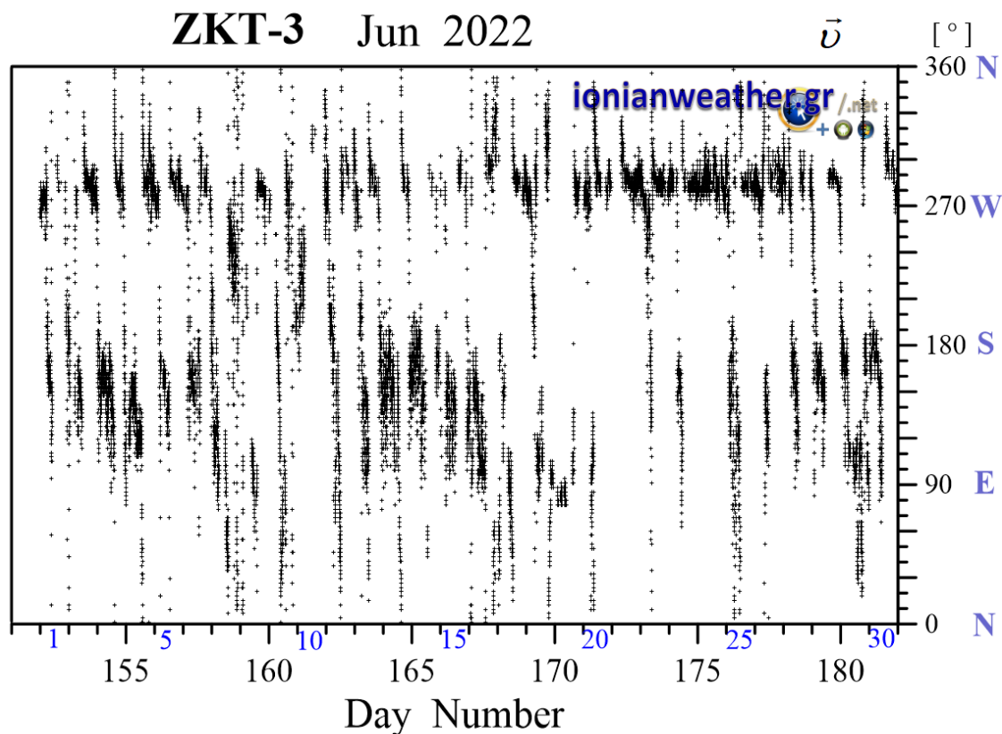
Εικόνα ZKT3-3: Μέση ανά λεπτό κατεύθυνση ανέμου Ιουνίου 2022 (κλίμακα αζιμουθίων δεξιά)
