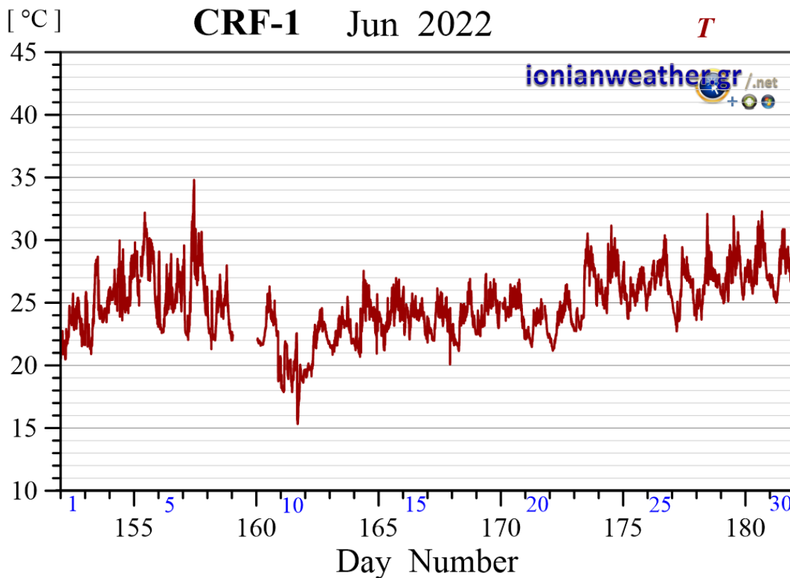
Εικόνα CRF1-4: Μέση ανά λεπτό θερμοκρασία αέρα Ιουνίου 2022.
