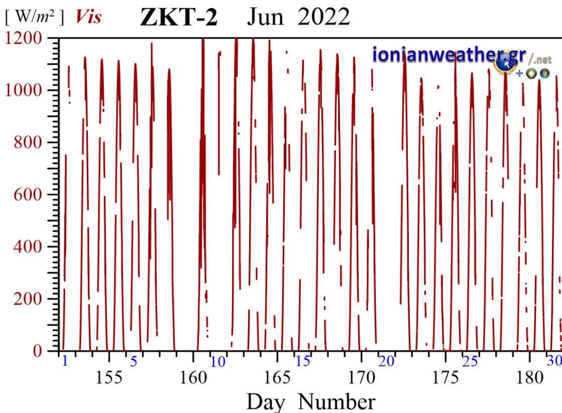
Εικόνα ZKT2-6: Μέση ανά λεπτό Ηλιακή ακτινοβολία Ιουνίου 2022 στην οπτική και εγγύς υπέρυθρη περιοχή.
