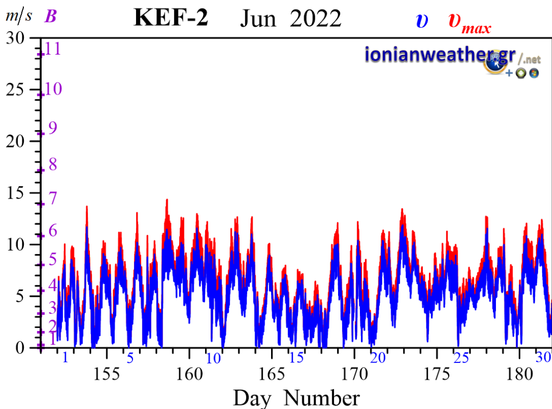
Εικόνα ΚΕF2-2: Μέση ανά λεπτό ταχύτητα ανέμου (m/s, γαλάζιο) και ριπή ανέμου (κόκκινο) Ιουνίου 2022. Κλίμακα ταχυτήτων αριστερά σε m/s και Beaufort.
