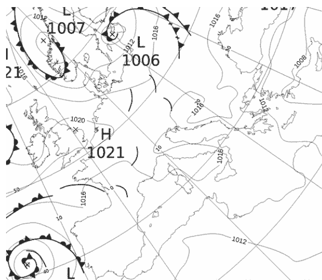
Εικόνα 3.1-2: MSLP 2 June 2022 00UTC
