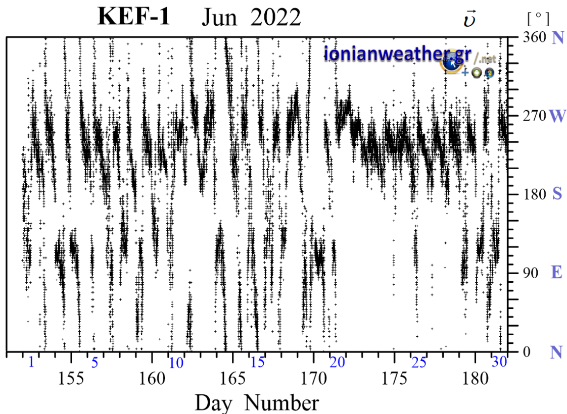
Εικόνα KEF1-3: Μέση ανά λεπτό κατεύθυνση ανέμου Ιουνίου 2022 (κλίμακα αζιμουθίων δεξιά)
