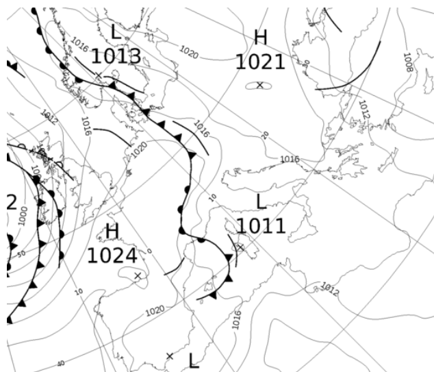
Εικόνα 3.1-28: MSLP 28 June 2022 00UTC
