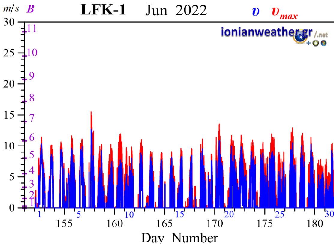
Εικόνα LFK1-2: Μέση ανά λεπτό ταχύτητα ανέμου (m/s, γαλάζιο) και ριπή ανέμου (κόκκινο) Ιουνίου 2022. Κλίμακα ταχυτήτων αριστερά σε m/s και Beaufort.
