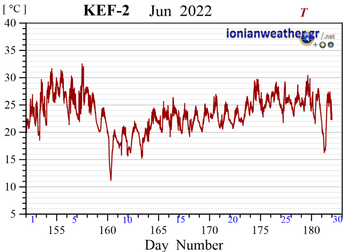
Εικόνα KEF2-4 Μέση ανά λεπτό θερμοκρασία αέρα Ιουνίου 2022.
