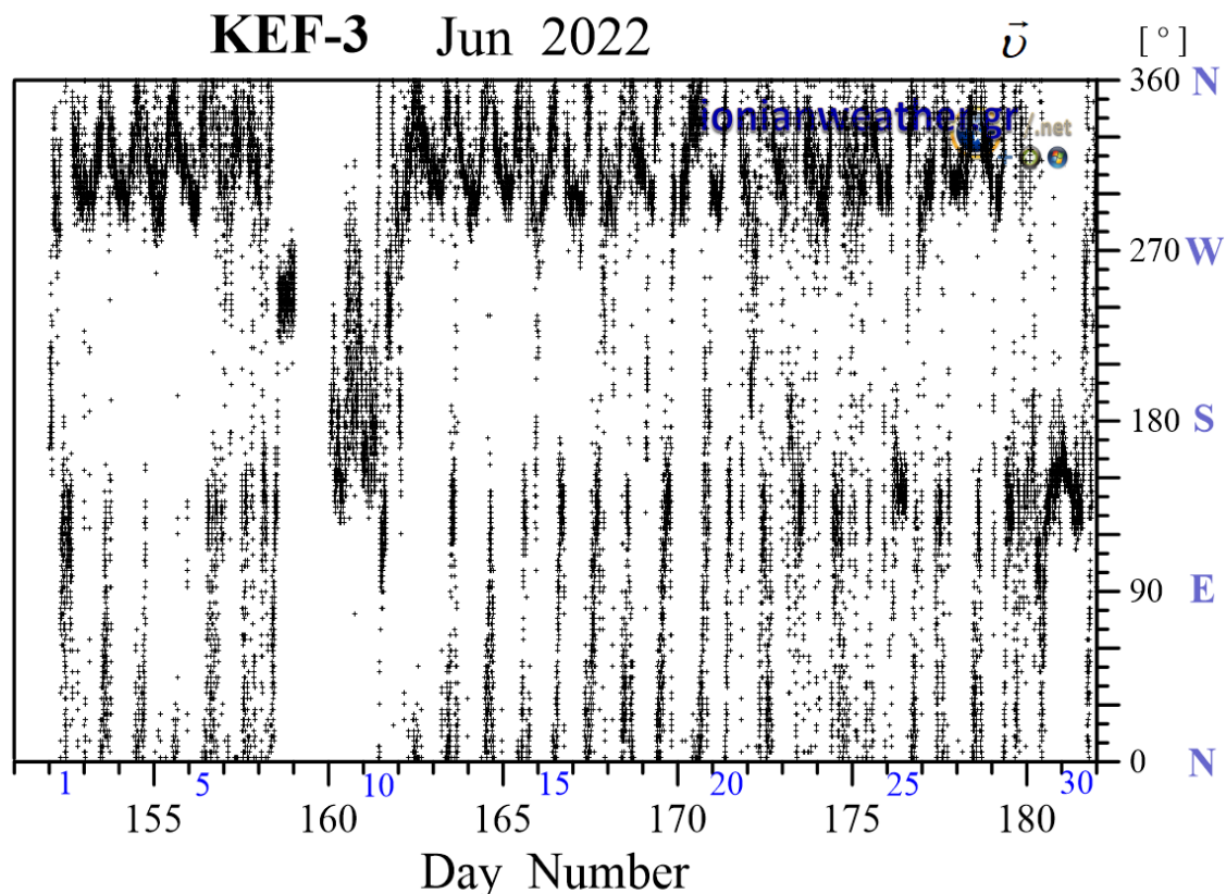
Εικόνα KEF3-3: Μέση ανά λεπτό κατεύθυνση ανέμου Ιουνίου 2022 (κλίμακα αζιμουθίων δεξιά)
