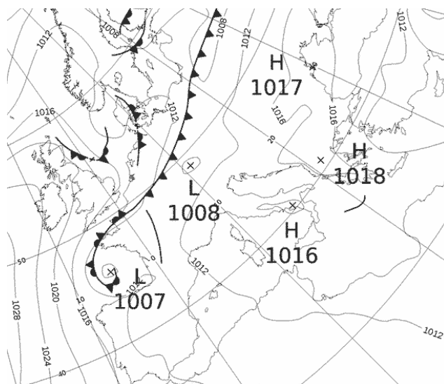
Εικόνα 3.1-20: MSLP 20 June 2022 00UTC
