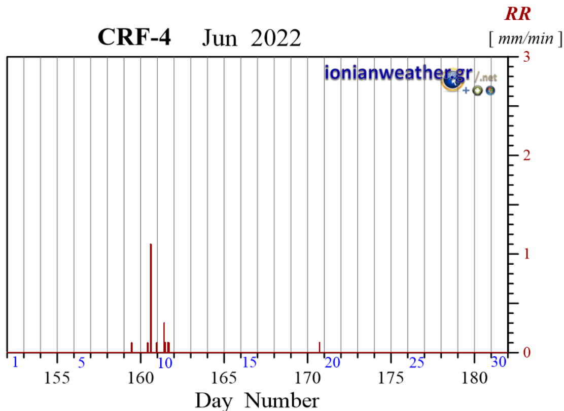
Εικόνα CRF4-1: Ανά λεπτό ρυθμός βροχόπτωσης (mm/min) Ιουνίου 2022.
