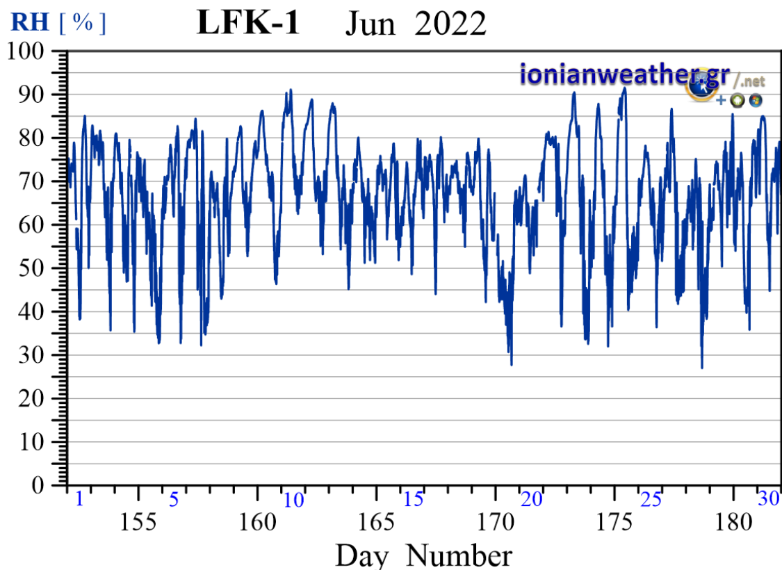
Εικόνα LFK1-5: Μέση ανά λεπτό σχετική υγρασία Ιουνίου 2022.
