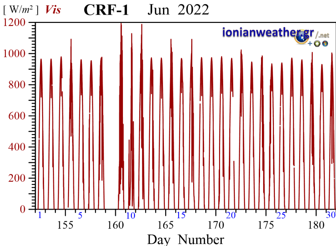
Εικόνα CRF1-7: Μέση ανά λεπτό Ηλιακή ακτινοβολία Ιουνίου 2022 στην οπτική και εγγύς υπέρυθρη περιοχή.
