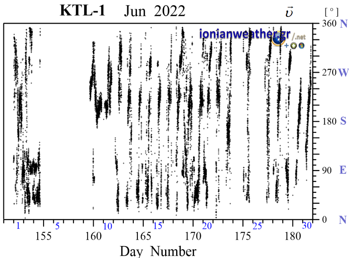
Εικόνα KTL1-3: Μέση ανά λεπτό κατεύθυνση ανέμου Ιουνίου 2022 (κλίμακα αζιμουθίων δεξιά)
