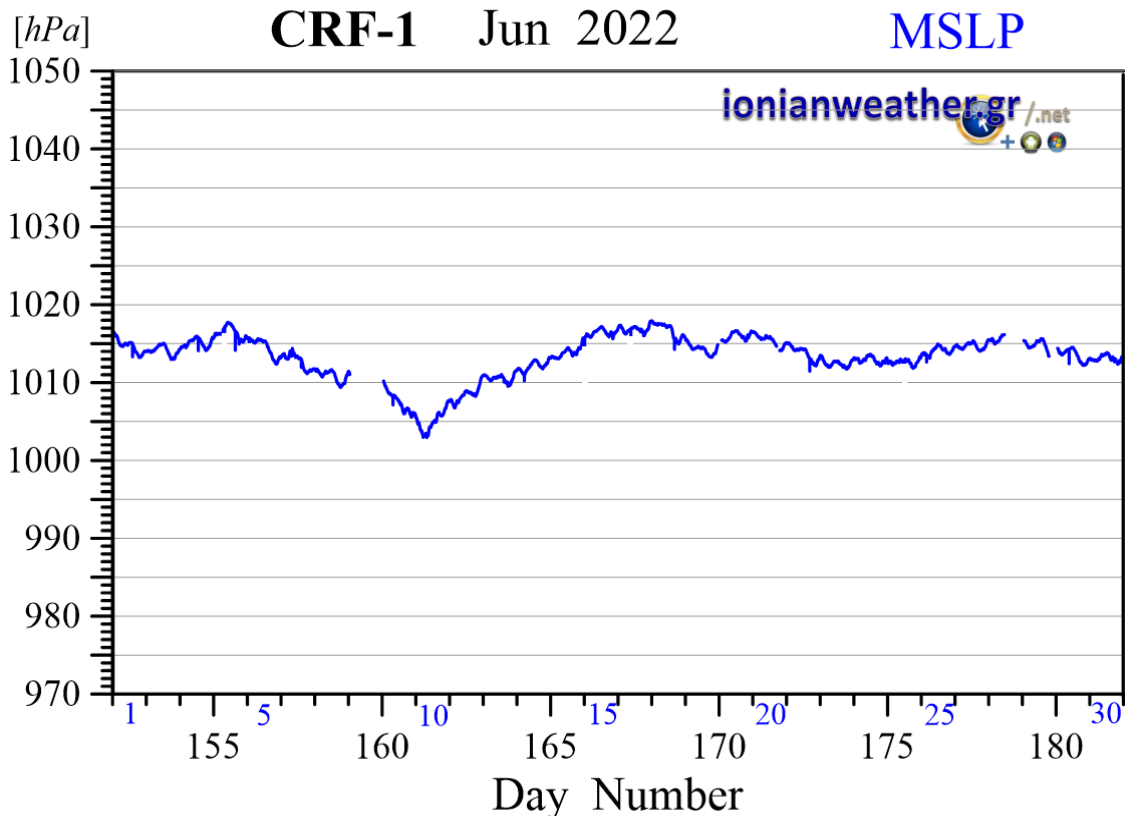
Εικόνα CRF1-6: Μέση ανά λεπτό βαρομετρική πίεση Ιουνίου 2022 ανηγμένη στην επιφάνεια της θάλασσας.
