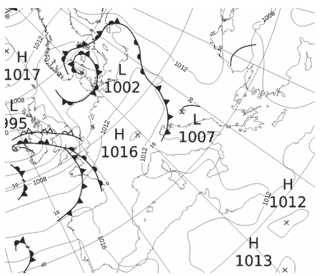
Εικόνα 3.1-8: MSLP 8 June 2022 00UTC
