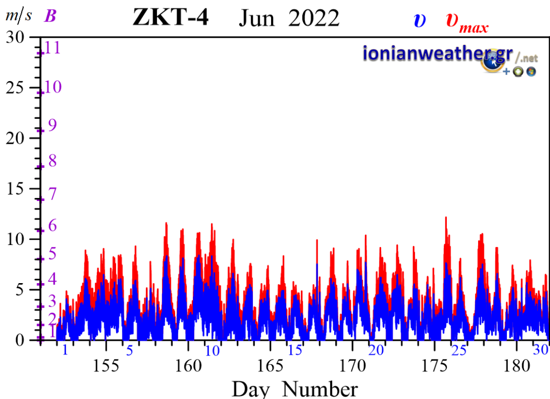
Εικόνα ZKT4-2: Μέση ανά λεπτό ταχύτητα ανέμου (m/s, γαλάζιο) και ριπή ανέμου (κόκκινο) Ιουνίου 2022. Κλίμακα ταχυτήτων αριστερά σε m/s και Beaufort.
