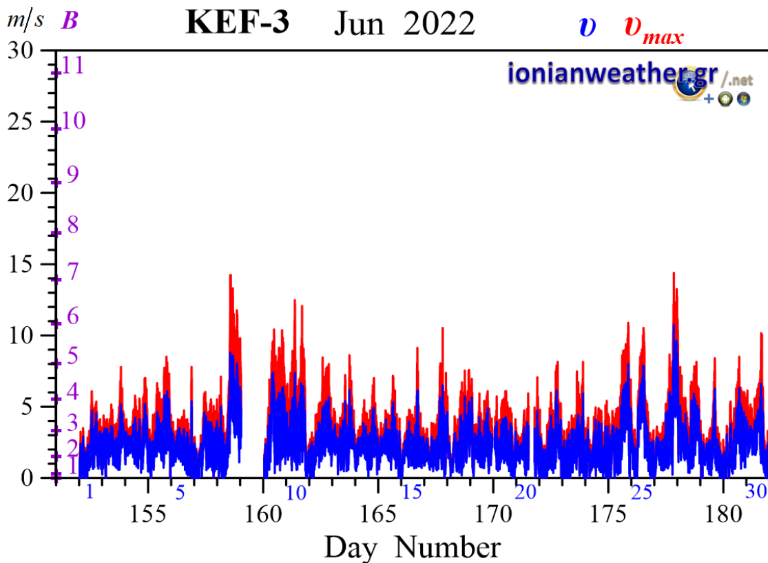
Εικόνα KEF3-2: Μέση ανά λεπτό ταχύτητα ανέμου ( m/s , γαλάζιο) και ριπή ανέμου (κόκκινο) Ιουνίου 2022. Κλίμακα ταχυτήτων αριστερά σε m/s και Beaufort .
