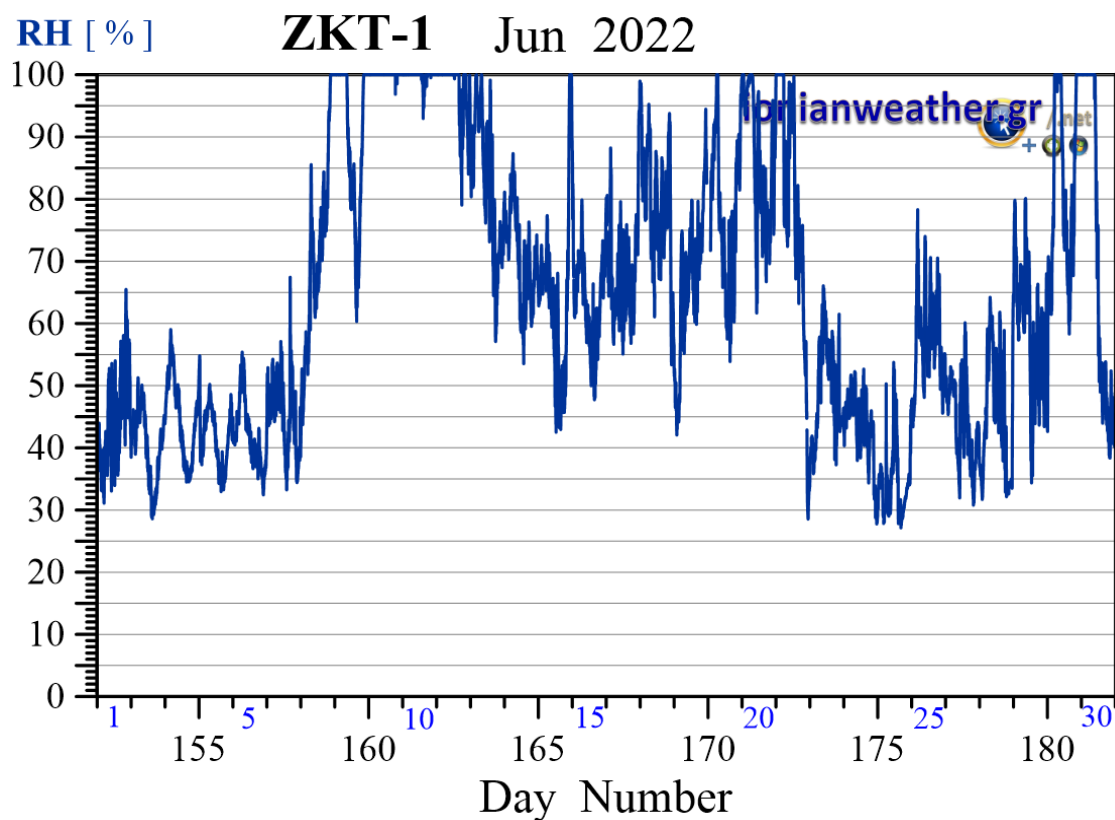
Εικόνα ZKT1-5: Μέση ανά λεπτό σχετική υγρασία Ιουνίου 2022.
