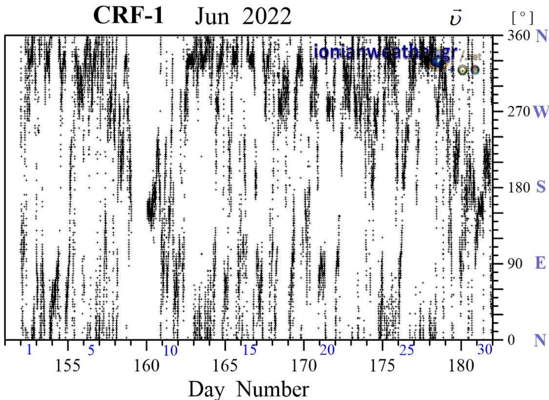
Εικόνα CRF1-3: Μέση ανά λεπτό κατεύθυνση ανέμου Ιουνίου 2022 (κλίμακα αζιμουθίων δεξιά)
