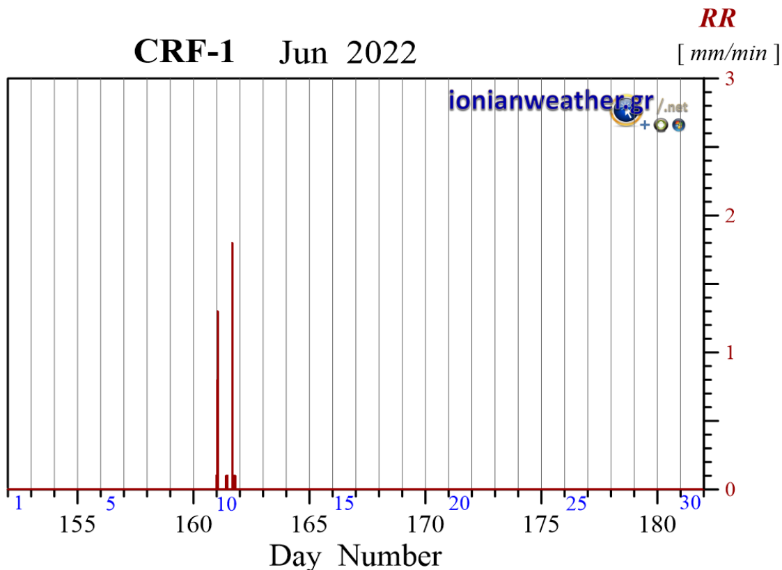
Εικόνα CRF1-1: Ανά λεπτό ρυθμός βροχόπτωσης ( mm/min ) Ιουνίου 2022.
