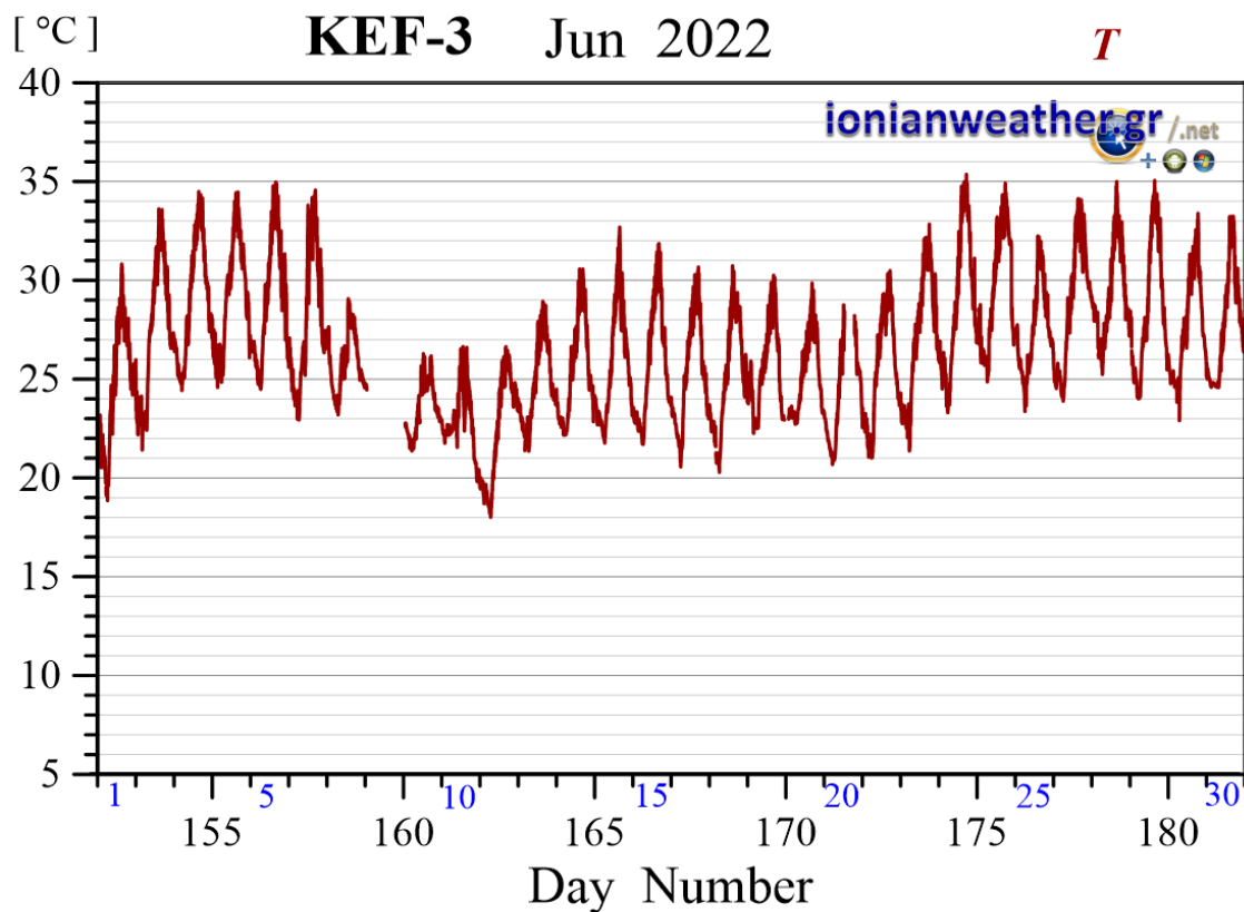
Εικόνα KEF3-4: Μέση ανά λεπτό θερμοκρασία αέρα Ιουνίου 2022.
