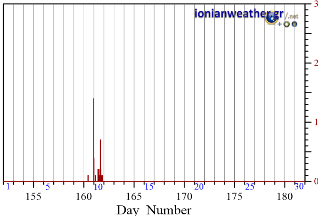
Εικόνα CRF2-1: Ανά λεπτό ρυθμός βροχόπτωσης (mm/min) Ιουνίου 2022.
