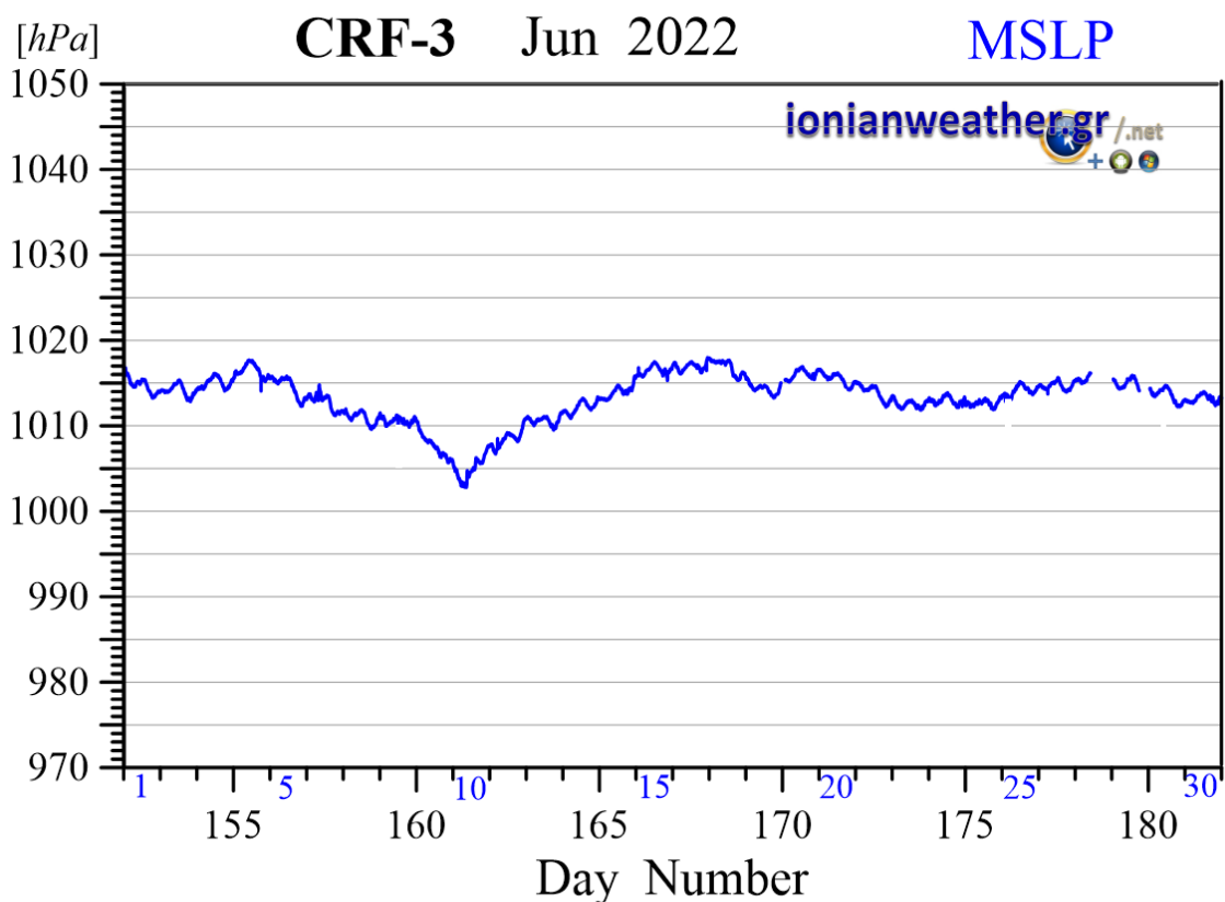
Εικόνα CRF3-6: Μέση ανά λεπτό βαρομετρική πίεση Ιουνίου 2022 ανηγμένη στην επιφάνεια της θάλασσας.
