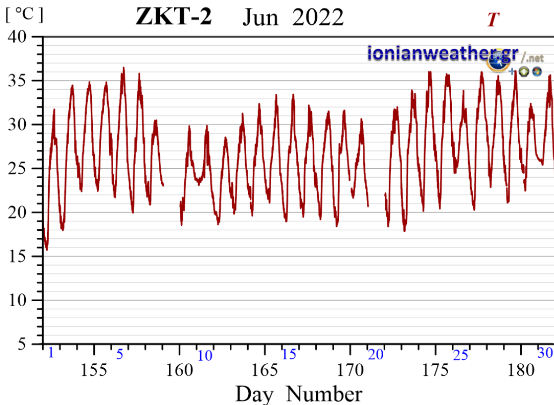
Εικόνα ZKT2-4: Μέση ανά λεπτό θερμοκρασία αέρα Ιουνίου 2022.
