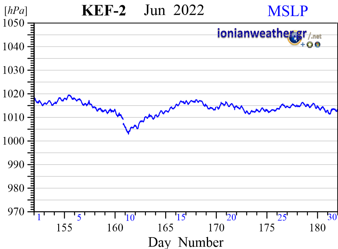
Εικόνα KEF2-6: Μέση ανά λεπτό βαρομετρική πίεση Ιουνίου 2022 ανηγμένη στην επιφάνεια της θάλασσας.
