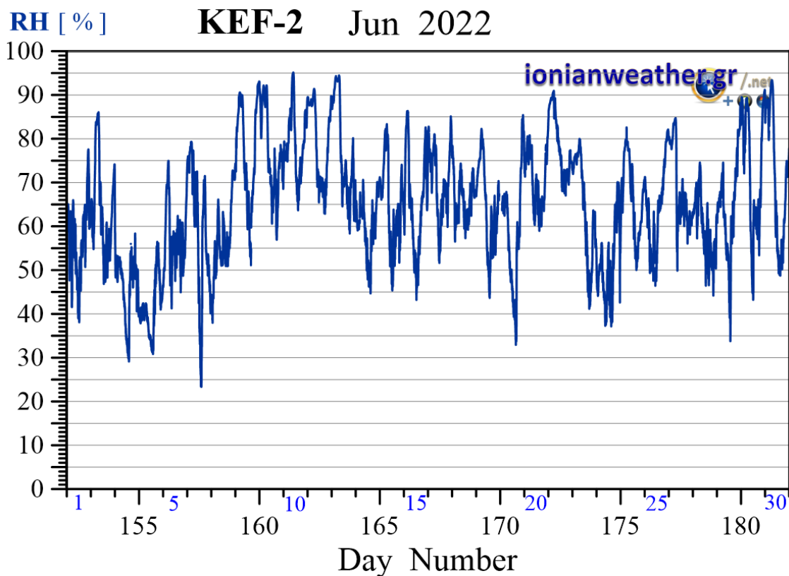
Εικόνα KEF2-5: Μέση ανά λεπτό σχετική υγρασία Ιουνίου 2022.
