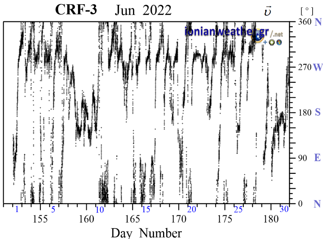
Εικόνα CRF3-3: Μέση ανά λεπτό κατεύθυνση ανέμου Ιουνίου 2022 (κλίμακα αζιμουθίων δεξιά)
