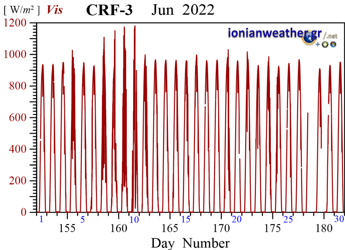
Εικόνα CRF3-7: Μέση ανά λεπτό Ηλιακή ακτινοβολία Ιουνίου 2022 στην οπτική και εγγύς υπέρυθρη περιοχή.
