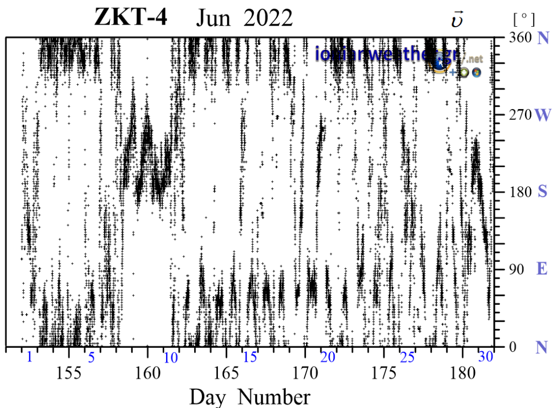
Εικόνα ZKT4-3: Μέση ανά λεπτό κατεύθυνση ανέμου Ιουνίου 2022 (κλίμακα αζιμουθίων δεξιά)
