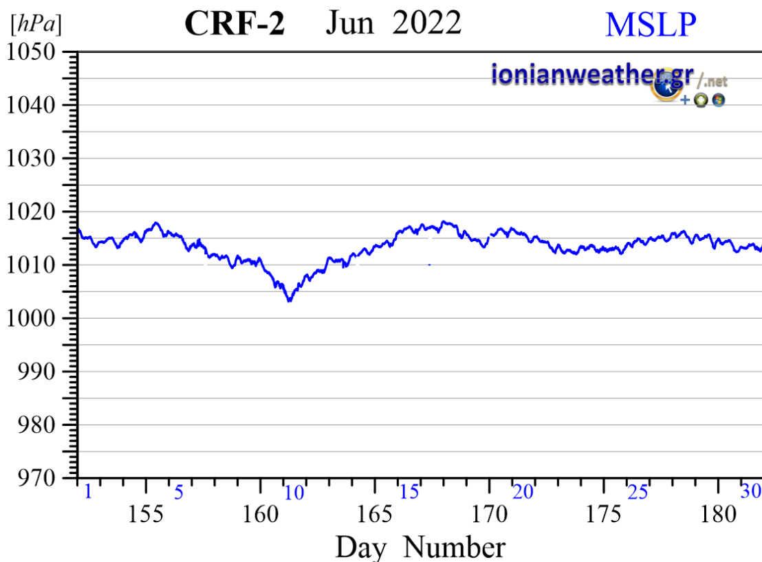
Εικόνα CRF2-6: Μέση ανά λεπτό βαρομετρική πίεση Ιουνίου 2022 ανηγμένη στην επιφάνεια της θάλασσας.
