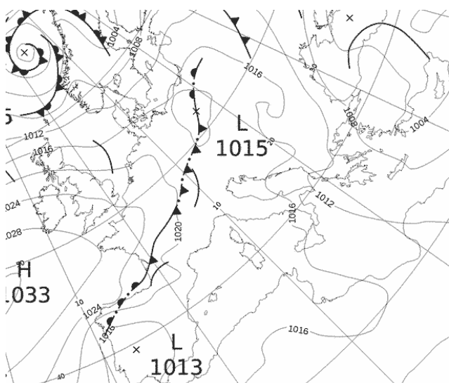
Εικόνα 3.1-13: MSLP 13 June 2022 00UTC
