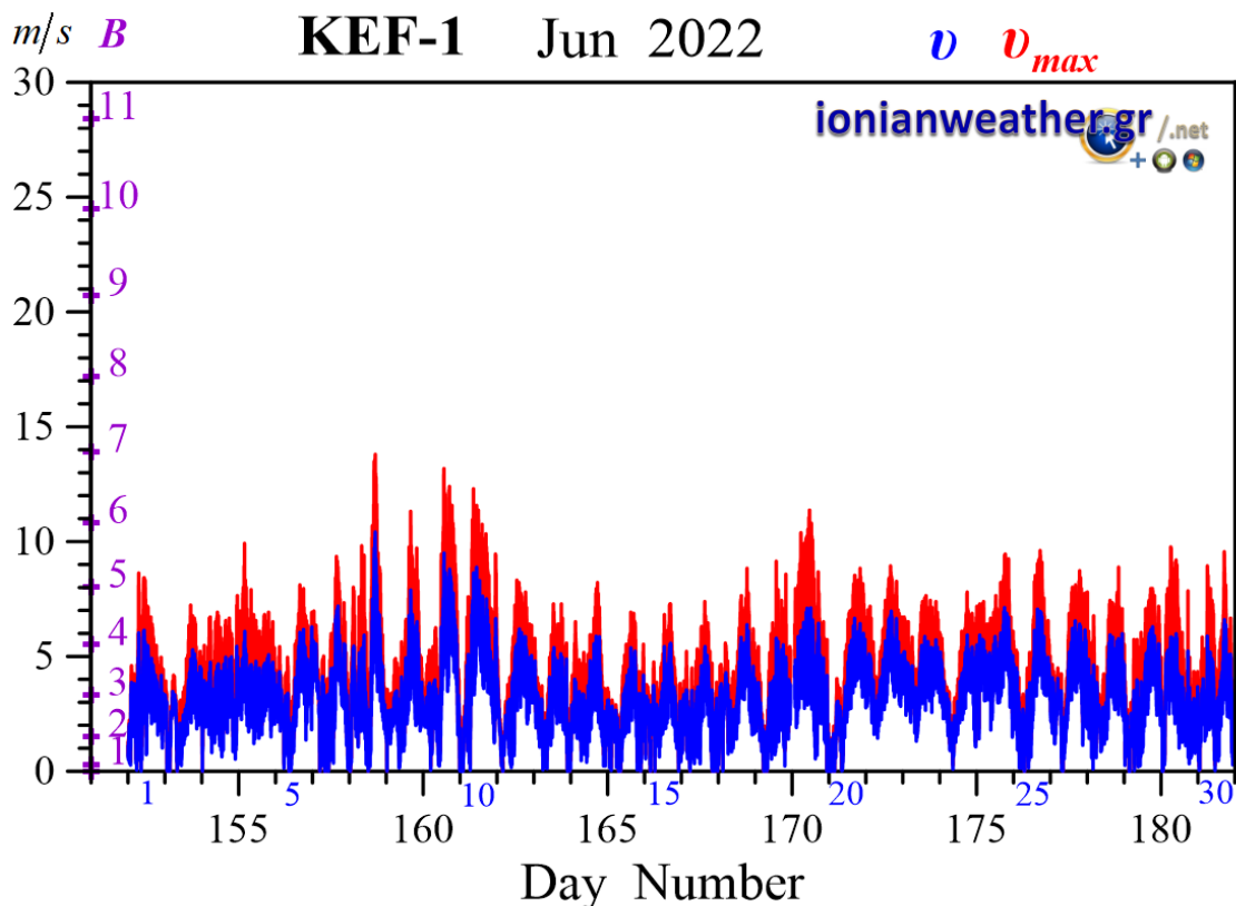
Εικόνα KEF1-2: Μέση ανά λεπτό ταχύτητα ανέμου (m/s, γαλάζιο) και ριπή ανέμου (κόκκινο) Ιουνίου 2022. Κλίμακα ταχυτήτων αριστερά σε m/s και Beaufort.
