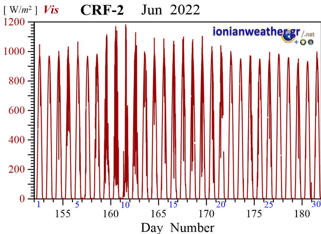
Εικόνα CRF2-7: Μέση ανά λεπτό Ηλιακή ακτινοβολία Ιουνίου 2022 στην οπτική περιοχή.
