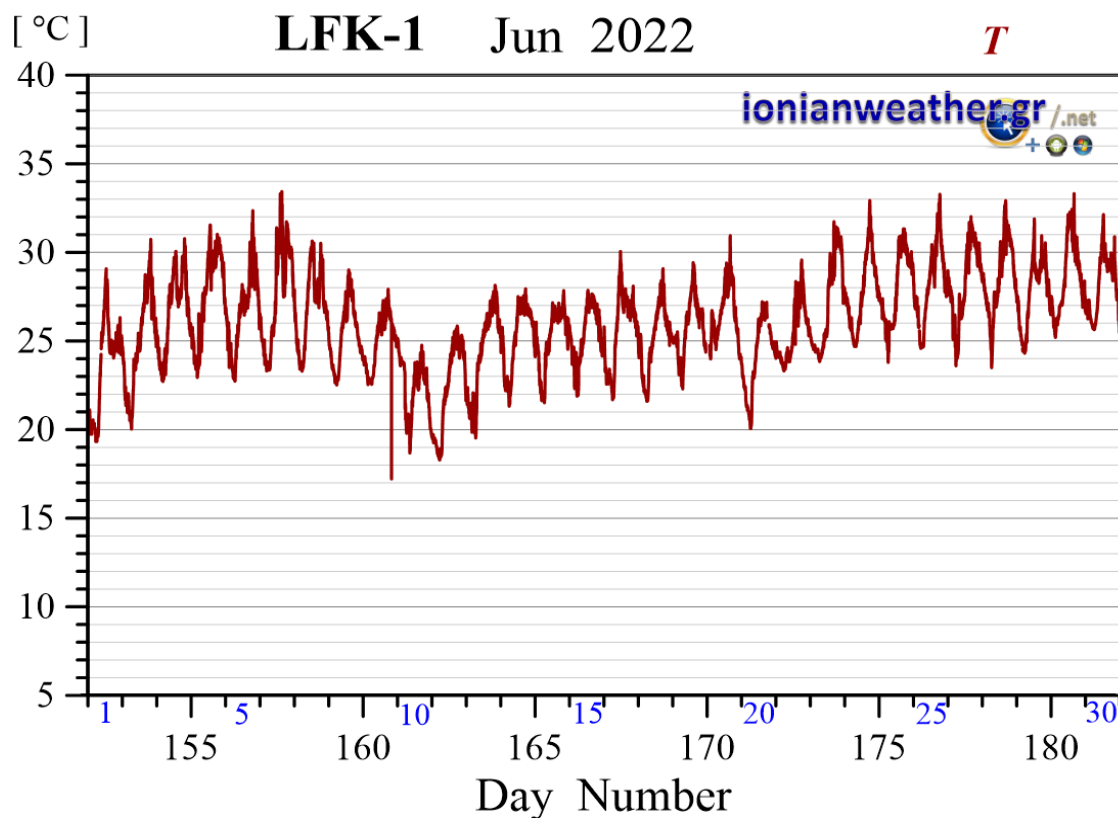
Εικόνα LFK1-4: Μέση ανά λεπτό θερμοκρασία αέρα Ιουνίου 2022.
