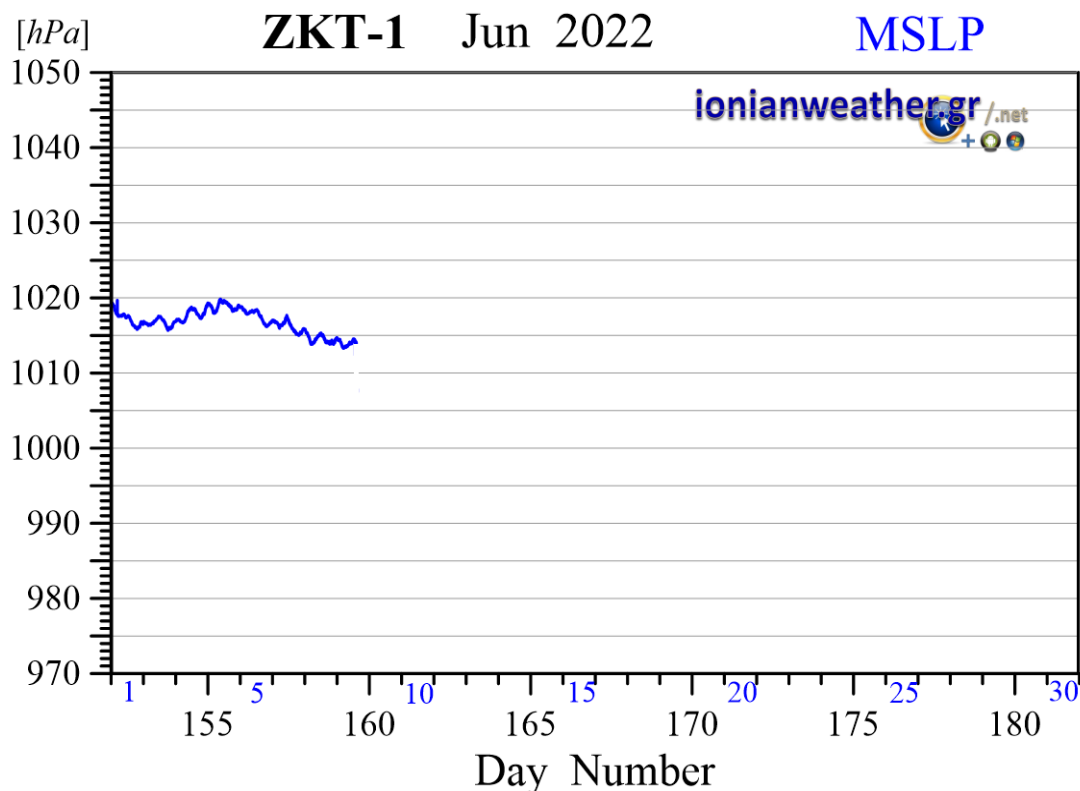
Εικόνα ZKT1-6: Μέση ανά λεπτό βαρομετρική πίεση Ιουνίου 2022 ανηγμένη στην επιφάνεια της θάλασσας.
