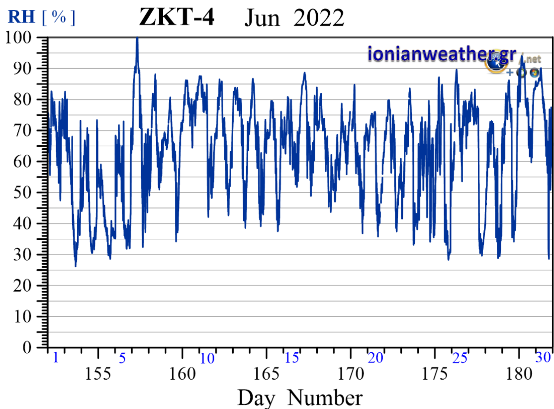
Εικόνα ZKT4-5: Μέση ανά λεπτό σχετική υγρασία Ιουνίου 2022.
