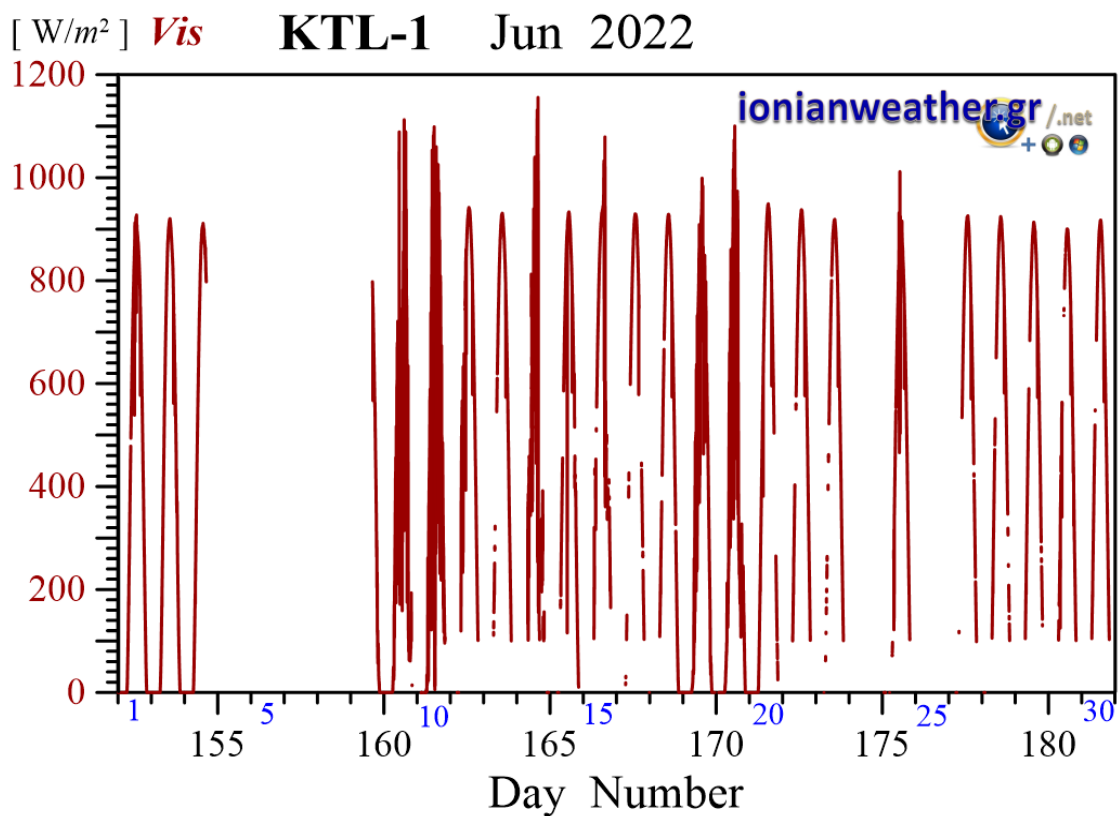
Εικόνα KTL1-7: Μέση ανά λεπτό Ηλιακή ακτινοβολία Ιουνίου 2022 στην οπτική και εγγύς υπέρυθρη περιοχή.
