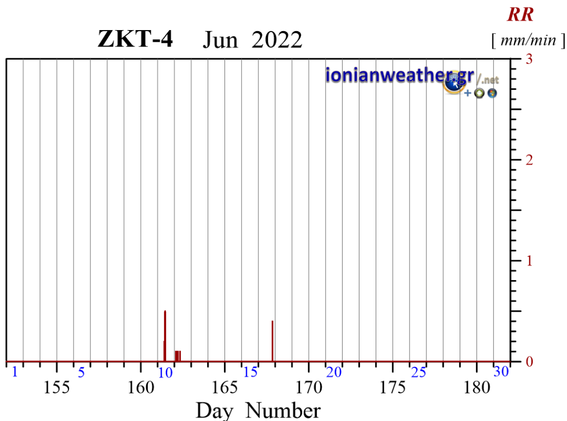
Εικόνα ZKT4-1: Ανά λεπτό ρυθμός βροχόπτωσης (mm/min) Ιουνίου 2022.
