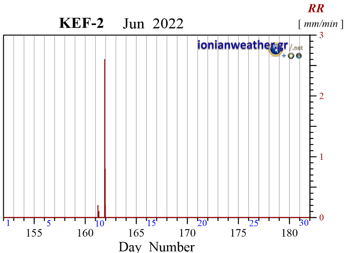
Εικόνα ΚΕF2-1: Ανά λεπτό ρυθμός βροχόπτωσης (mm/min) Ιουνίου 2022.
