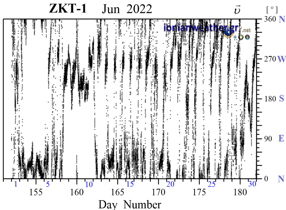
Εικόνα ZKT1-3: Μέση ανά λεπτό κατεύθυνση ανέμου Ιουνίου 2022 (κλίμακα αζιμουθίων δεξιά)
