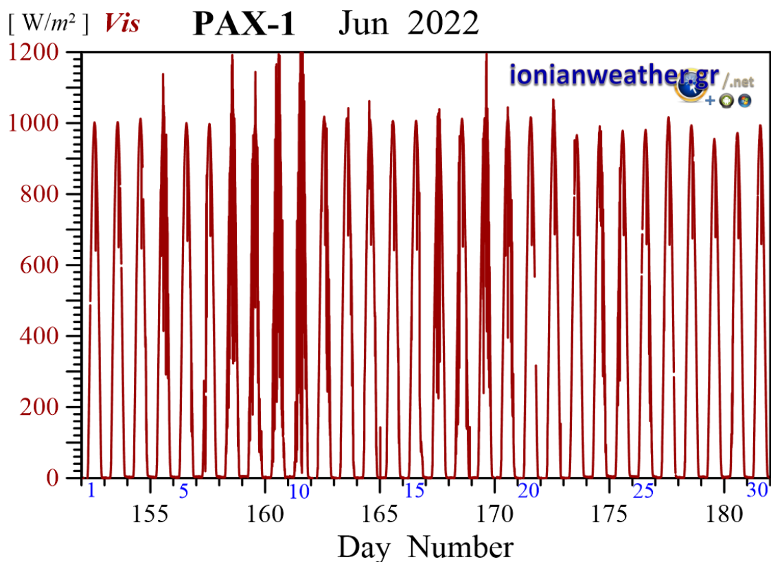
Εικόνα PAX1-6: Μέση ανά λεπτό Ηλιακή ακτινοβολία Ιουνίου 2022 στην οπτική και εγγύς υπέρυθρη περιοχή.
